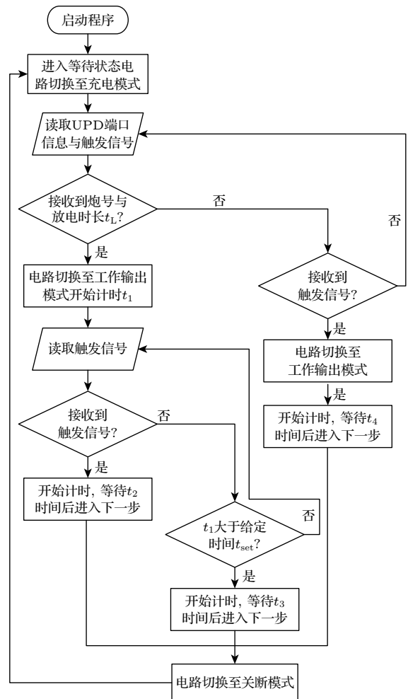
图 2 电容充放电控制电路的自动控制流程图
