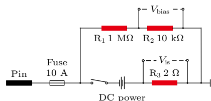
图 12 限制器探针的离子饱和流测量电路
