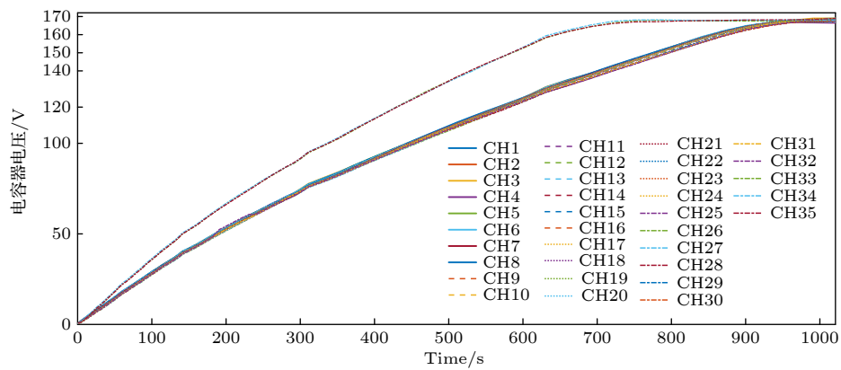
图 8 电容器充电曲线, 其中通道 1—32, 使用 1 台直流电源同时为 4 台电容器充电; 通道 33—35, 使用 1 台直流电源为 3 台电容器充电
