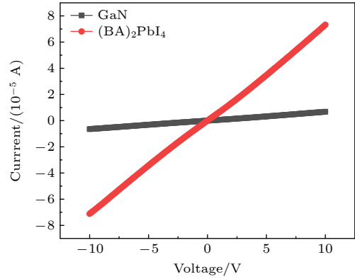
图 4 GaN 和 (BA) 2 PbI 4 的电流-电压特性曲线.
