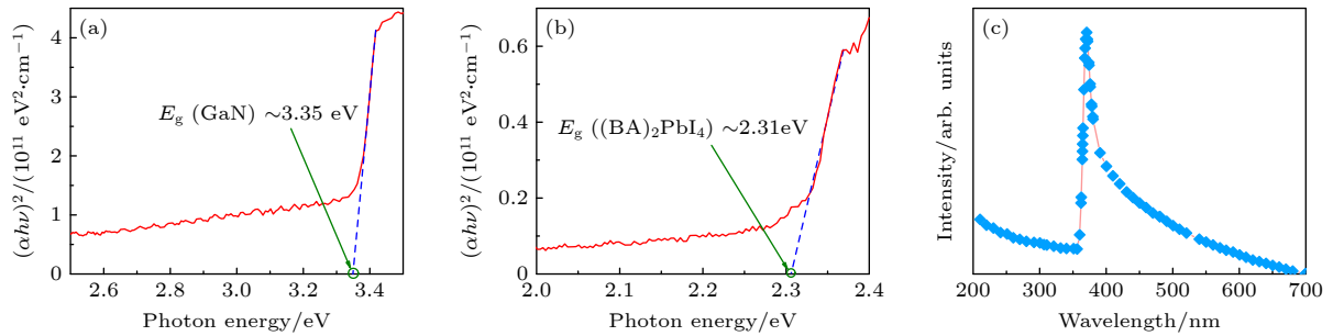
图 2 (a), (b) (\alpha h\nu)^2 与 (h\nu) 的拟合函数图; (c) GaN/(BA) 2 PbI 4 异质结的紫外-可见光响应谱
