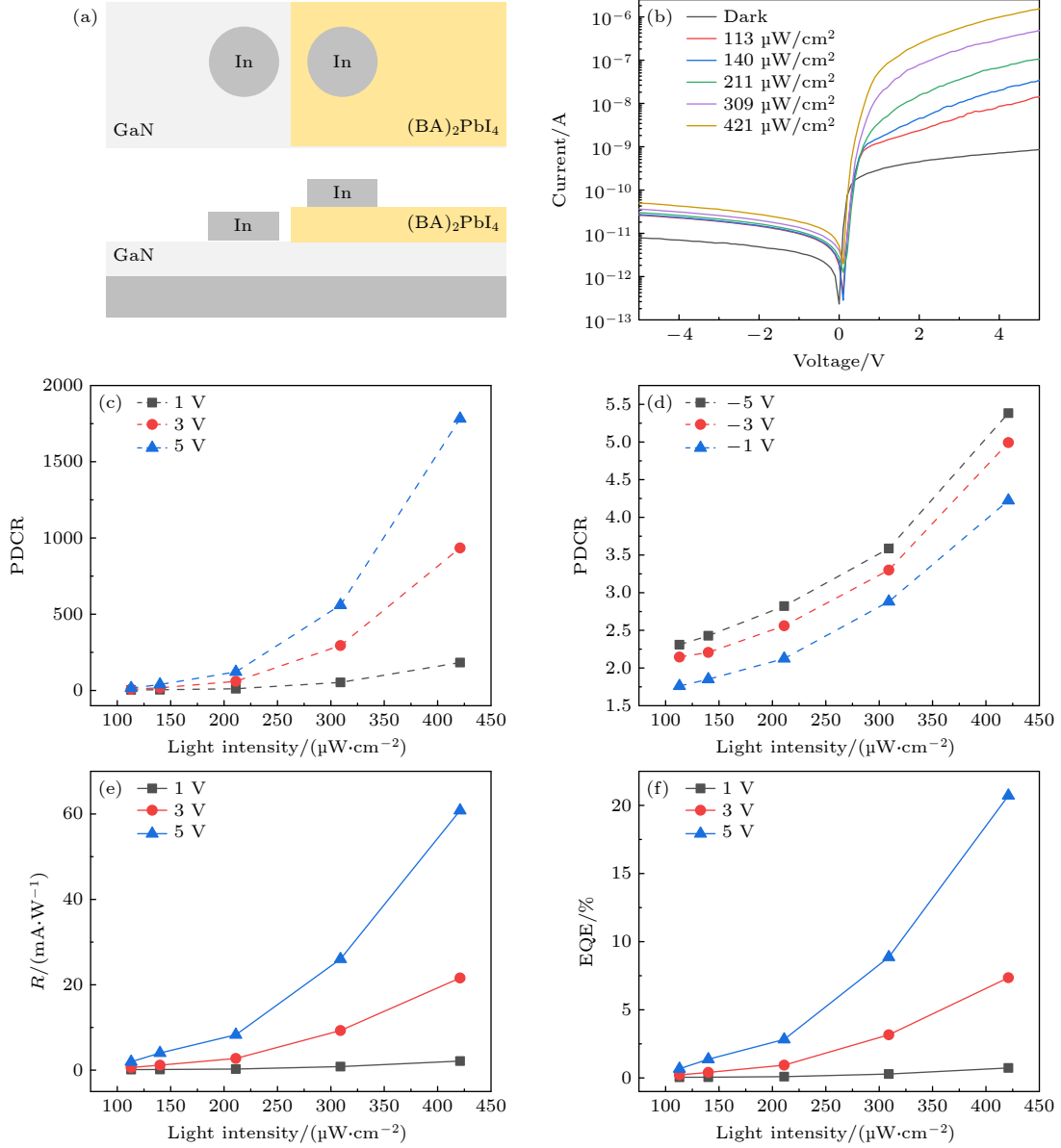
图 3 (a) GaN/(BA) 2 PbI 4 异质结光电探测器示意图; (b) 异质结光电探测器在黑暗中和不同强度的 365 nm 紫外光照下的对数坐标 I - V 特性曲线; (c), (d) 在不同电压下探测器的 PDCR 和光强度的关系; (e), (f) 在不同电压下响应度 ( R ) 和外部量子效率 (EQE) 与光强度的关系
