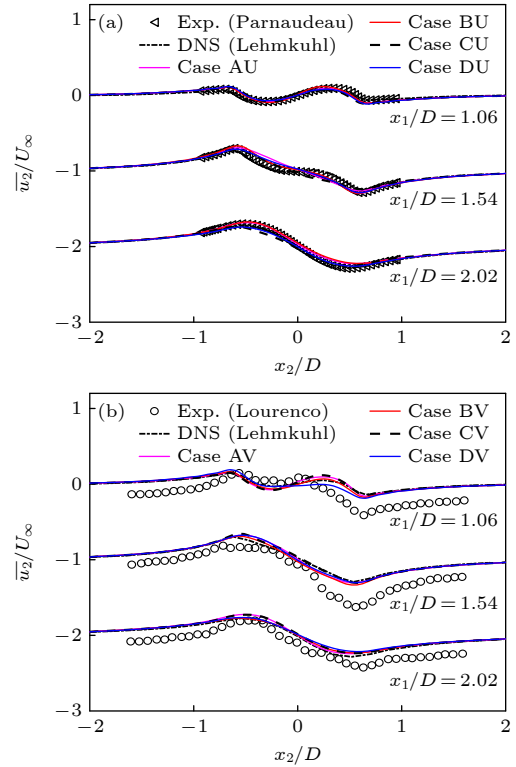
图 7 圆柱后方不同站位处平均横向速度剖面特性
