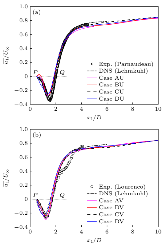
图 5 沿尾流中心线平均流向速度剖面特性
