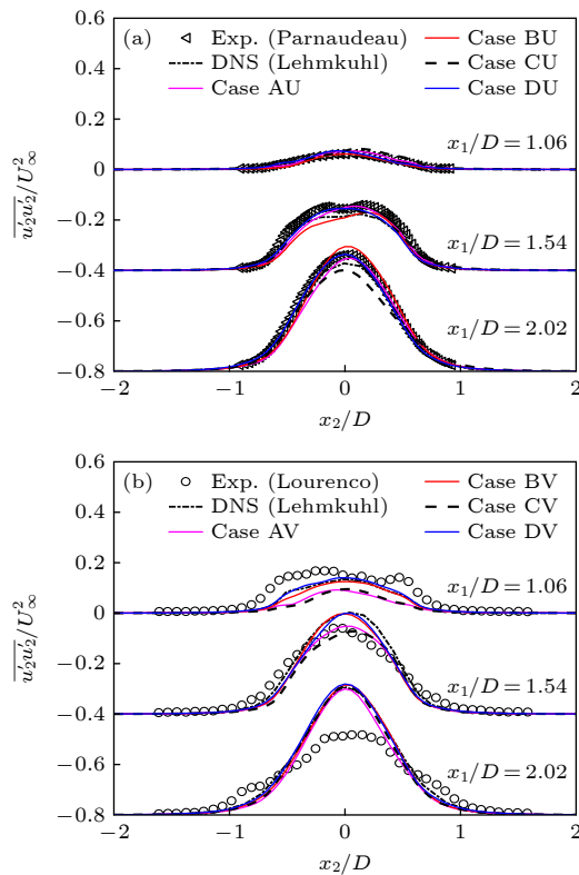
图 9 圆柱后方不同站位处各向同性横向雷诺应力剖面特性
