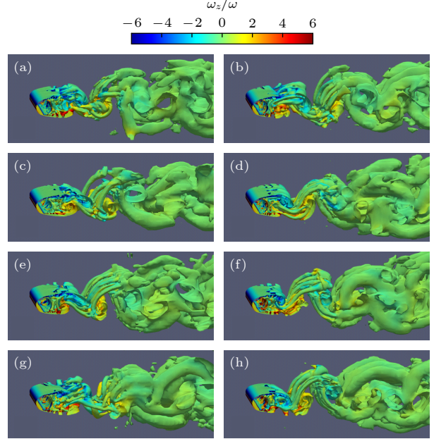
图 15 在 Case AU—DU (左) 和 Case AV—DV (右) 工况下, 圆柱绕流展向三维涡量云图
