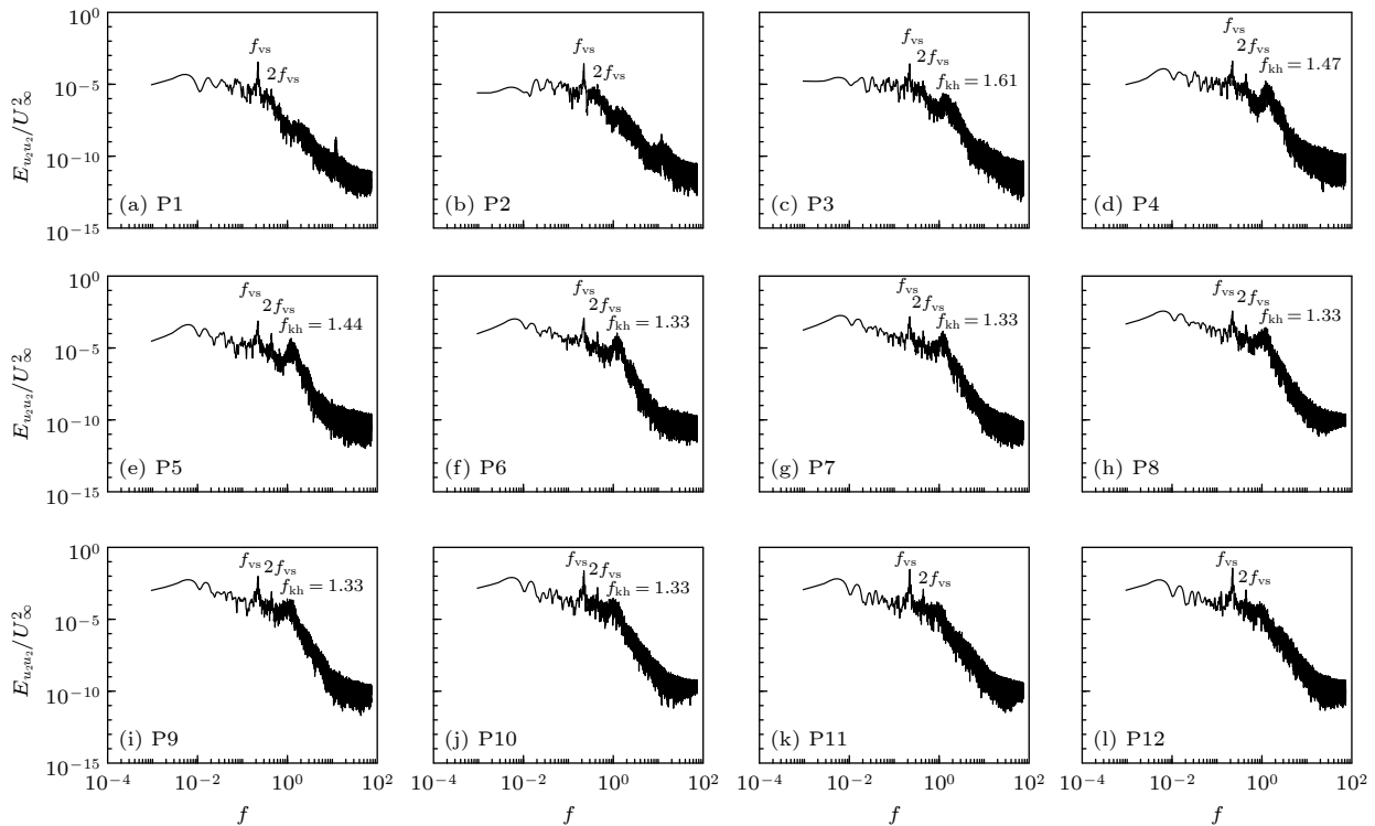
图 11 在 Case CU 工况下,在 P1—P12 监测点处横向脉动速度的 Lomb 谱
