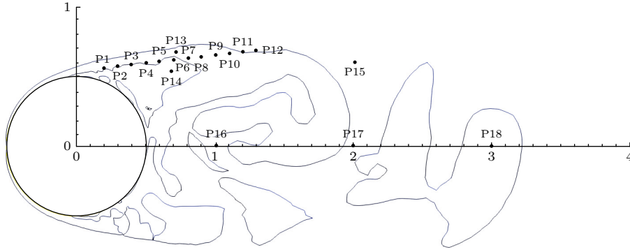
图 3 剪切层小尺度 K-H 不稳定性结构监测点分布
