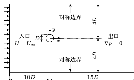
图 1 计算区域设置
