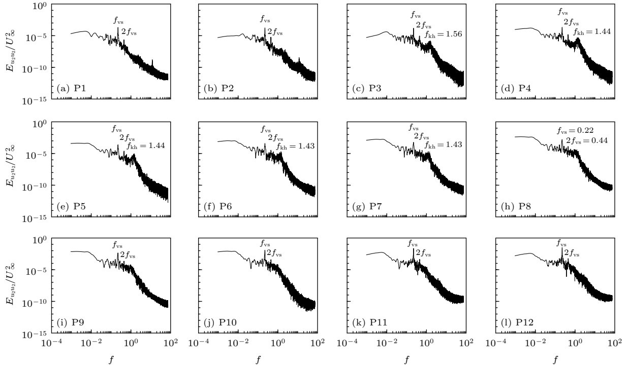
图 12 在 Case CV 工况下, 在 P1—P12 监测点处横向脉动速度的 Lomb 谱
