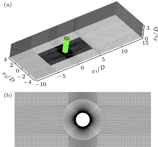
图 2 计算网格剖面
