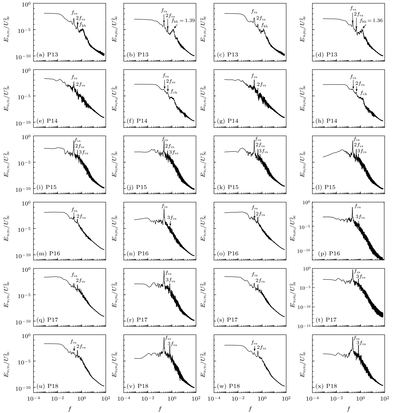
图 13 在 Case CU (第 1 和第 2 列) 和 Case CV (第 3 和第 4 列) 工况下, 在 P13—P18 监测点处流向 (第 1 和第 3 列) 及横向 (第 2 和第 4 列) 脉动速度的 Lomb 谱
