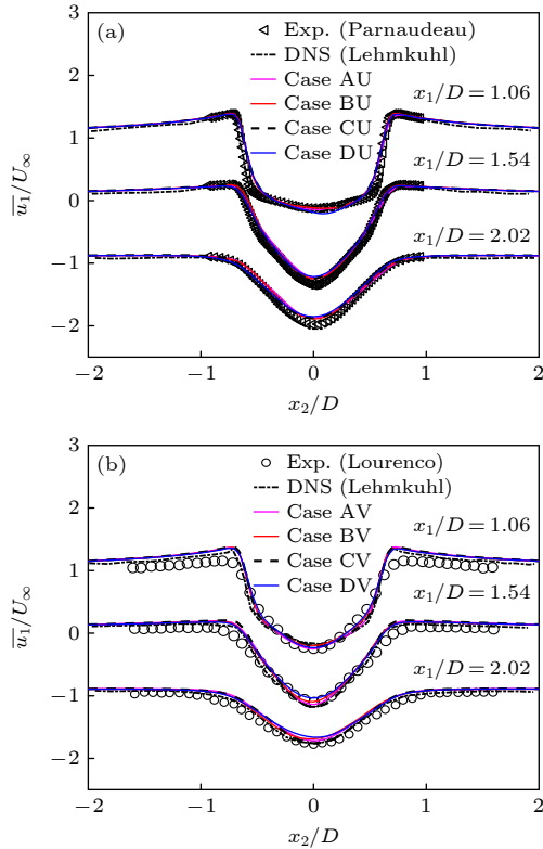
图 6 圆柱后方不同站位处平均流向速度剖面特性
