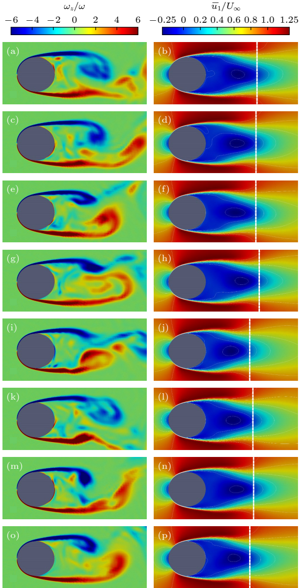
图 14 在 Case AU—DU(前 4 行) 和 Case AV—DV(后 4 行) 工况下, 圆柱绕流涡量(左) 及流向速度(右) 云图
