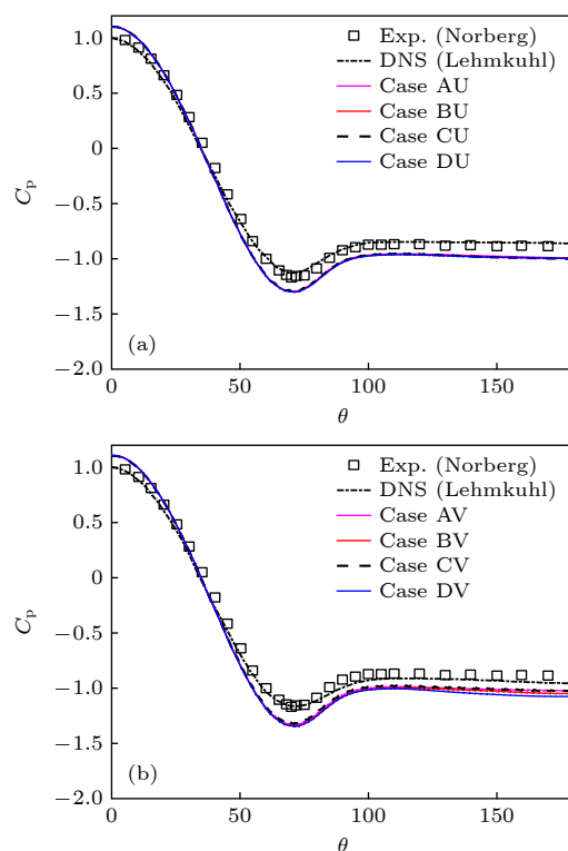
图 4 圆柱表面周向压力系数 C_p 分布特性
