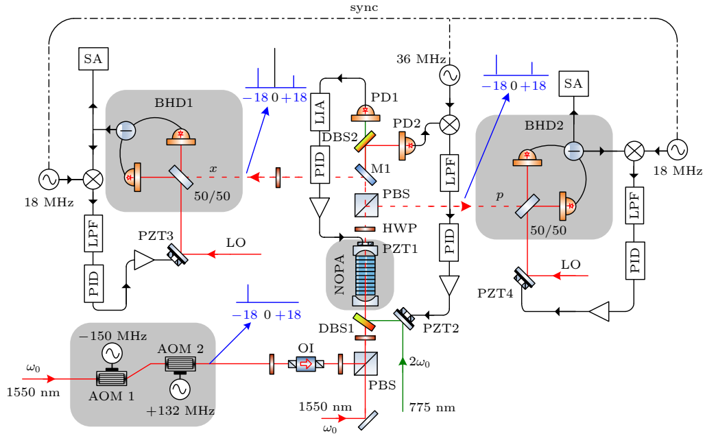
OI, 光学隔离器; DBS, 双色分束镜; PBS, 偏振分束器; HWP, 半波片; PZT, 压电陶瓷; PD, 光电探测器; SA, 频谱分析仪; LIA, 锁相放大器; PID, 比例积分微分器; LFP, 低通滤波器; \otimes , 混频器; \Delta , 高压放大器; sync, 同步触发
