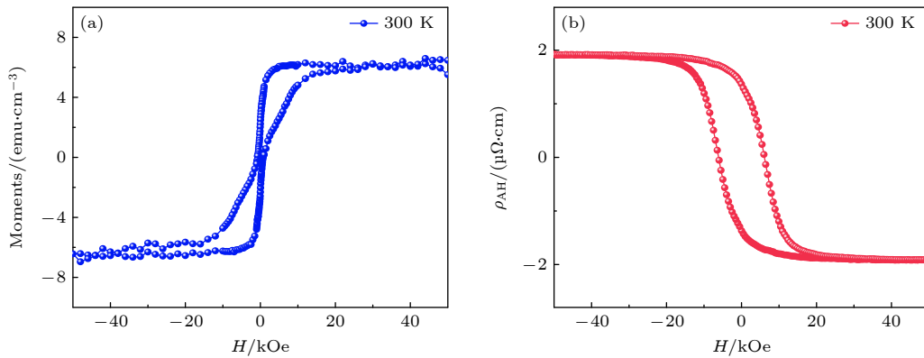
图 2 室温下 \text{Mn}_3\text{Sn} 薄膜的 (a) 垂直磁化曲线, 以及 (b) AHE 电阻率随磁场的变化
