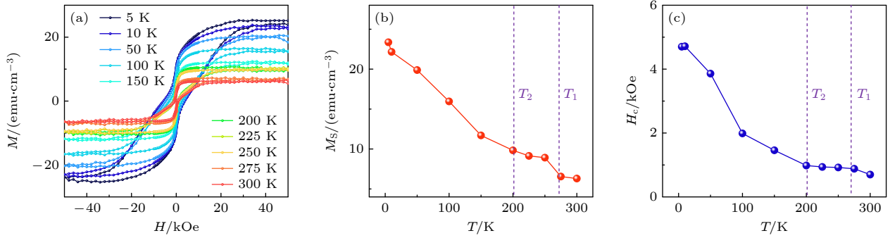
图 3 (a) 不同温度下的磁化曲线 ( 1 \text{ emu}/\text{cm}^3 = 10^3 \text{ A}/\text{m} ); (b) 饱和磁化强度 ( M_s ) 和 (c) 矫顽力 ( H_c ) 随温度的变化
