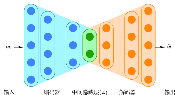
图 1 自编码器神经网络架构示意图, 蓝色部分表示编码器 (encoder) 函数 f(\cdot) , 橙色部分表示解码器 (decoder) 函数 g(\cdot) , 维度最低绿色表示中间隐藏层 ( z ). 对自编码器, 损失函数是输出 ( \tilde{x}_i ) 与输入 x_i 的差别的函数 (也可以加正则化项, 如参考文献 [58] (5) 式所示), 每一个输入数据点对应隐藏层空间的一个点
