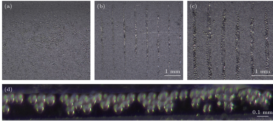
图 5 PS 微球操控实验效果图 (a) 当压电声子晶体板未加载电信号时 PS 微球的初始状态; (b) 当压电声子晶体板加载共振频率为 0.998 MHz 的电信号时 PS 微球的状态; (c) 加载共振频率为 1.072 MHz 的电信号时 PS 微球的状态; (d) 图 (c) 侧视图
