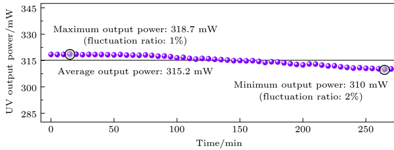
图 7 紫外 VECSEL 输出功率的稳定性
