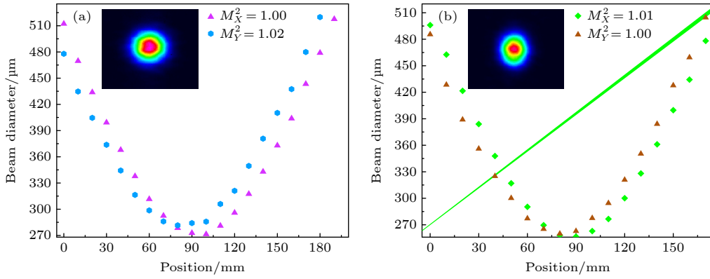
图 6 (a) 基频激光的光束质量 M^2 因子, 插图为光强的二维分布图; (b) 倍频激光的光束质量 M^2 因子, 插图为对应的二维光强分布图
