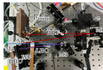
图 2 紫外 VECSEL 实物图
