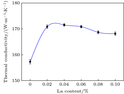
图 9 不同 La 添加量的 Al-7%Si-0.6%Fe 合金的热导率
