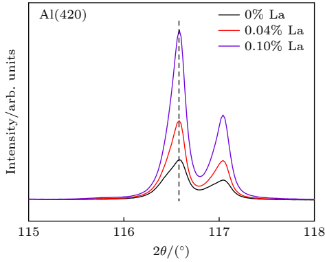
图 12 添加不同含量 La 时 \alpha -Al 相在高角度区间的 XRD 图谱 Fig. 12. XRD spectra of \alpha -Al phase in an elevation-angle zone with different addition of La.
