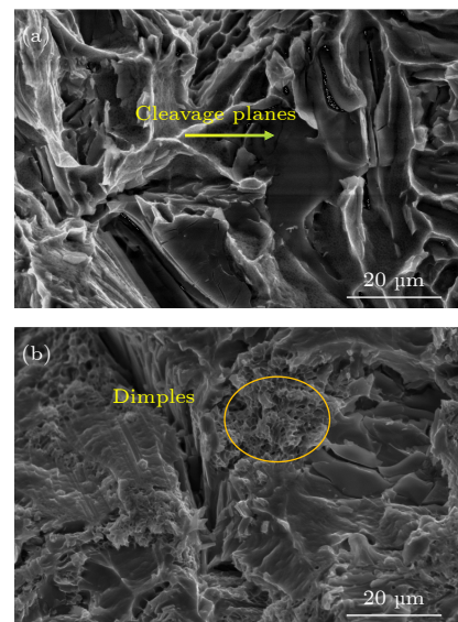
图 13 添加 La 前后 Al-7%Si-0.6%Fe-0.02Sr-0.024B 合金的拉伸断口形貌 (a) 未添加 La; (b) 添加 0.02% La Fig. 13. Tensile fracture morphology of Al-7%Si-0.6%Fe alloys before and after addition of La: (a) Without La; (b) add 0.02% La.
