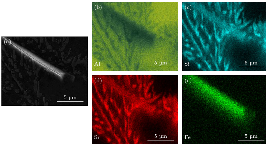
图 2 Al-7%Si-0.6%Fe-0.024%B-0.02%Sr 合金的 SEI 和 EDS 元素分布 (a) SEI; (b) Al; (c) Si; (d) Sr; (e) Fe. Fig. 2. SEI and EDS element distribution of Al-7%Si-0.6%Fe-0.024%B-0.02%Sr alloy: (a) SEI; (b) Al; (c) Si; (d) Sr; (e) Fe.
