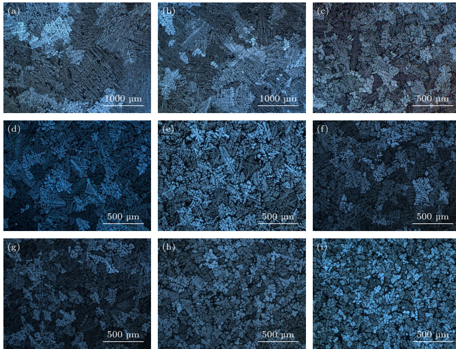
图 6 不同 Sr, B, La 添加量的 Al-7%Si-0.6%Fe 合金的 OM 图像 (a) 0; (b) 0.02% Sr; (c) 0.024% B; (d) 0.02% Sr 和 0.024% B; (e) 0.02% Sr, 0.024% B 和 0.02% La; (f) 0.02% Sr, 0.024% B 和 0.04% La; (g) 0.02% Sr, 0.024% B 和 0.06% La; (h) 0.02% Sr, 0.024% B 和 0.08% La; (i) 0.02% Sr, 0.024% B 和 0.10% La
