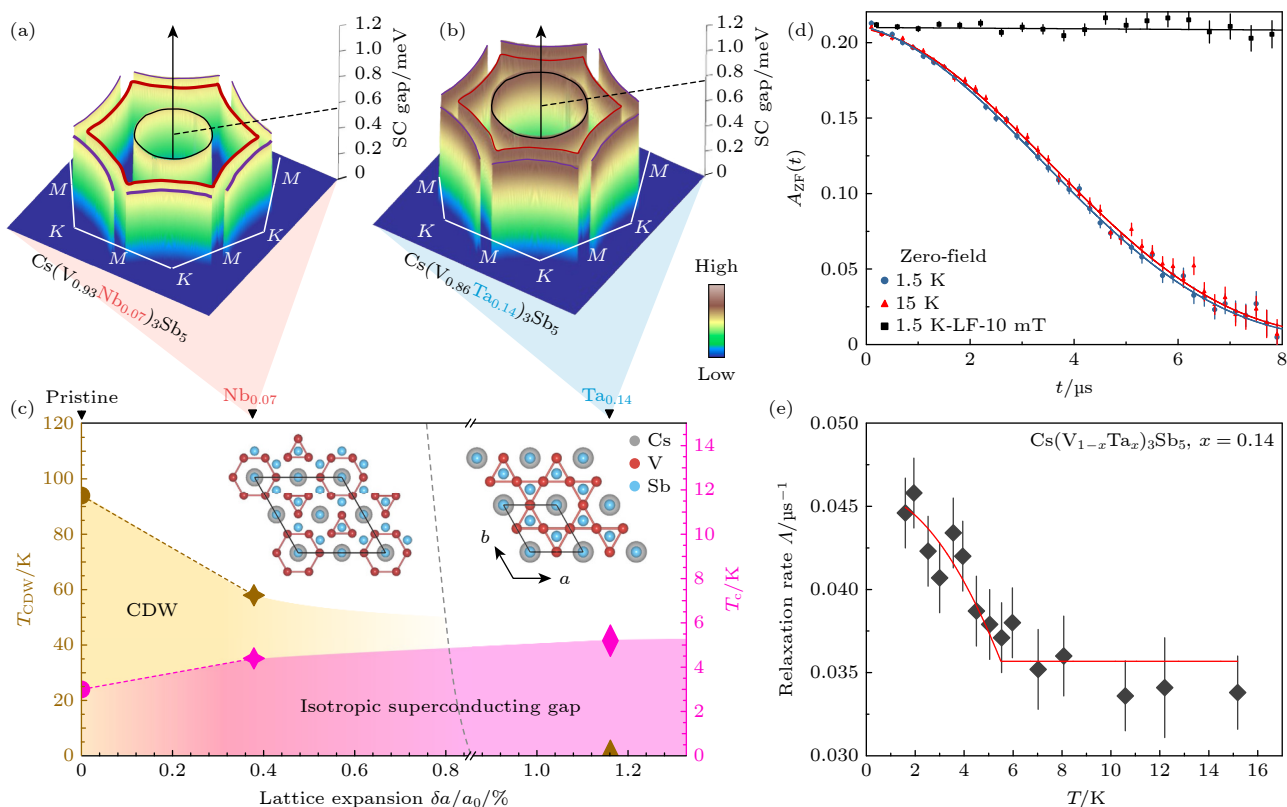
图 6 (a), (b) \text{Cs}(\text{V}_{0.93}\text{Nb}_{0.07})_3\text{Sb}_5 和 \text{Cs}(\text{V}_{0.86}\text{Ta}_{0.14})_3\text{Sb}_5 样品超导能隙的动量依赖关系示意图; (c) T_{\text{CDW}} , T_c 与晶格膨胀率的依赖关系的相图, 晶格膨胀率是由于化学替代引起的; (d) T_c 以下和以上 \text{Cs}(\text{V}_{0.86}\text{Ta}_{0.14})_3\text{Sb}_5 的零场 \mu\text{SR} 时间谱; (e) 零场 \mu 子自旋弛豫率在 T_c 附近的温度依赖关系; 表明在 CDW 被完全抑制时, \text{Cs}(\text{V}_{0.86}\text{Ta}_{0.14})_3\text{Sb}_5 的超导电性具有时间反演对称性破缺的特性 [47]
