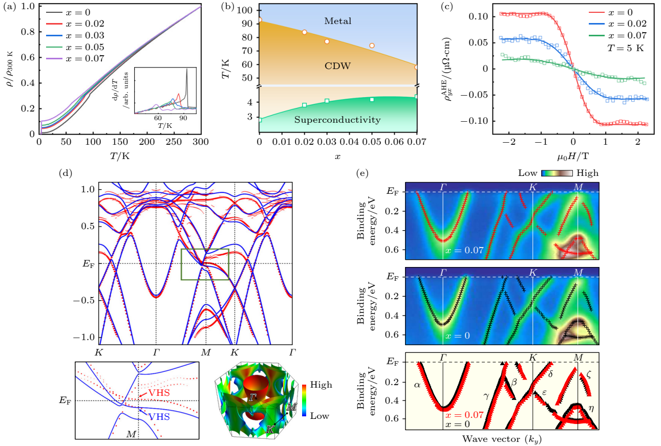
图 4 (a) 从 1.8 K 到 300 K, Cs(V_{1-x}Nb_x)_3Sb_5 的面内电阻率的温度依赖关系 [46] ; (b) Cs(V_{1-x}Nb_x)_3Sb_5 的相图, 表明了 CDW 和超导之间的竞争关系 [46] ; (c) 温度为 5 K 时, 去除线性正常霍尔背景后提取的反常霍尔电阻率 [46] ; (d) 第一性原理计算得到的 CsV_3Sb_5 和 Cs(V_{0.93}Nb_{0.07})_3Sb_5 的电子能带结构; (e) 上图和中图分别为 CsV_3Sb_5 和 Cs(V_{0.93}Nb_{0.07})_3Sb_5 沿 \Gamma KM 方向切割的 ARPES 强度图, 下图为拟合点的对比图 [49]
