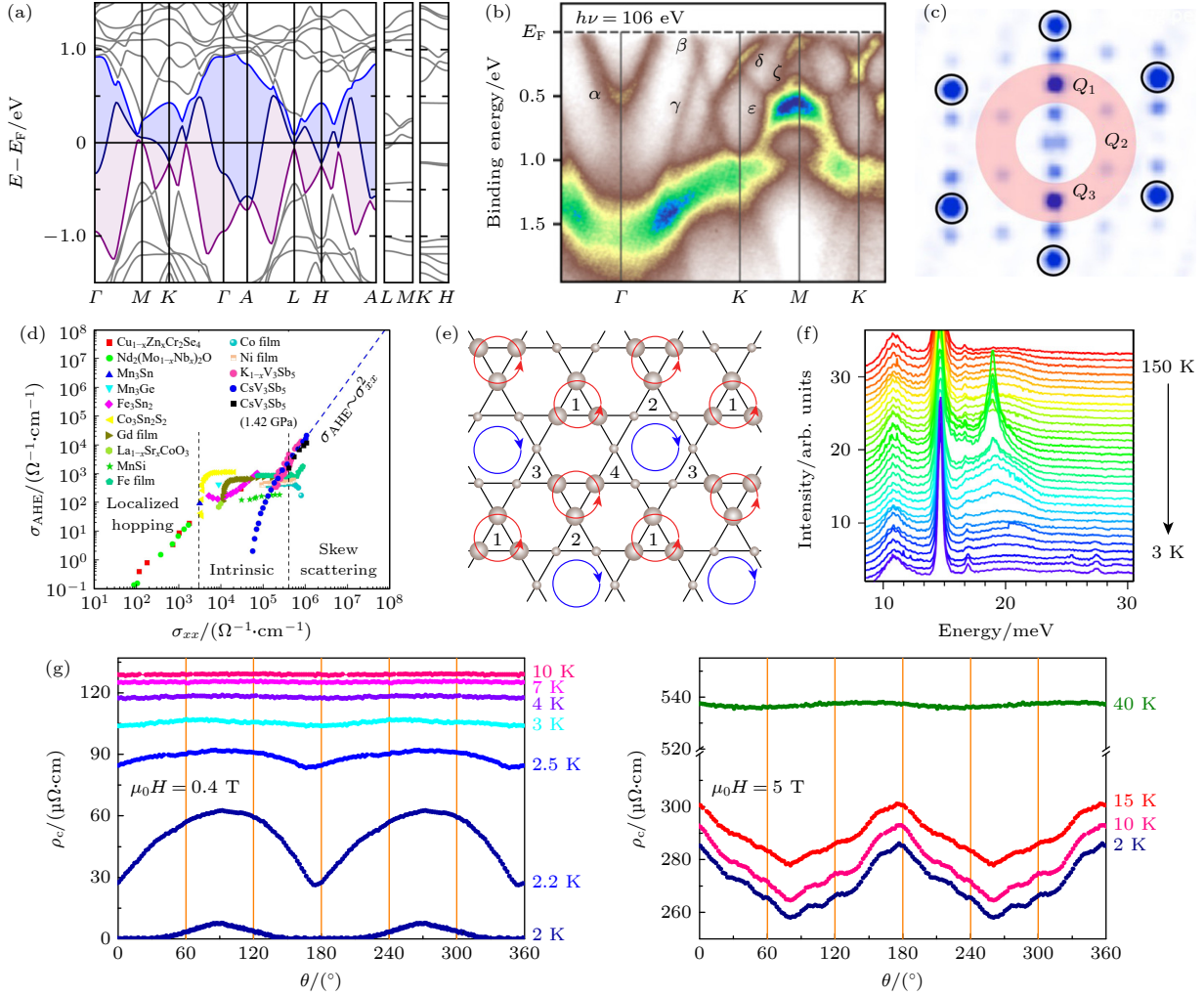
图 3 (a) DFT 计算的 \text{CsV}_3\text{Sb}_5 能带结构 [14] ; (b) ARPES 观察到的沿 \Gamma\text{KM} 方向的电子能带结构 [26] ; (c) Sb 表面形貌图的傅里叶变换, 显示 2\times 2 电荷序 (红色阴影区域) 和 1\times 4 电荷序 [33] ; (d) 覆盖从局域跃迁机制到偏斜散射机制的 \sigma_{\text{AHE}} 与 \sigma_{xx} 关系图, 包含多种材料与 \text{CsV}_3\text{Sb}_5 和 \text{K}_{1-x}\text{V}_3\text{Sb}_5 的对比 [37] ; (e) 手性磁通相的局域轨道磁矩分布及电荷分布 [40] ; (f) \text{KV}_3\text{Sb}_5 的拉曼光谱, 低温条件下在 25.4 meV 和 27.5 meV 时观察到两种新的声子模式 [45] ; (g) 外加 0.4 T 和 5 T 磁场时, 不同温度下 c 轴方向的电阻率随测量角度的依赖关系 [43]
