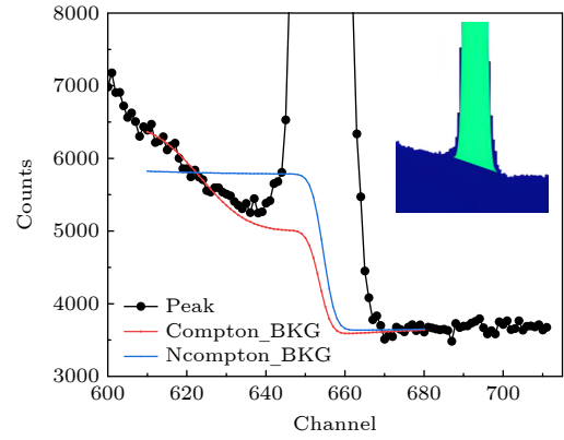
图 9 是否包含康普顿边缘部分本底拟合结果比较,其中插图为 GammaVision 处理效果
