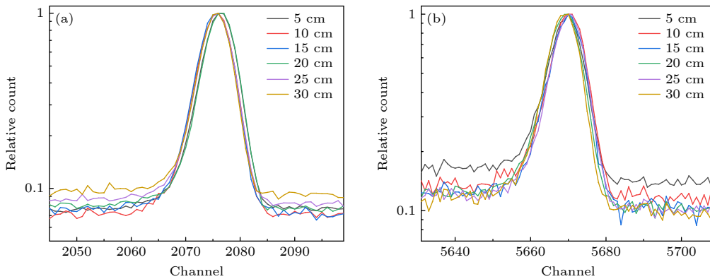
图 5 同轴 HPGe 探测器不同源距同一能量的特征 \gamma 射线峰峰形对比 (a) 443.965 keV 射线峰; (b) 1212.948 keV 射线峰
