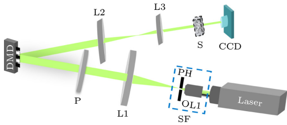
图 4 实验装置
