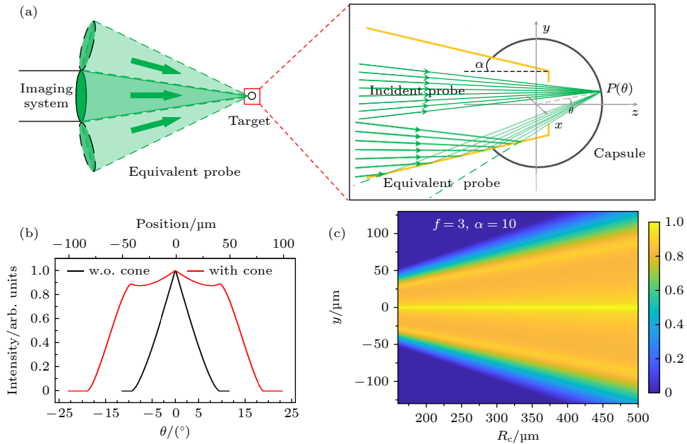
图 2 (a) 利用 keyhole 锥壁反射效应时球形反射面的 VISAR 诊断示意图; (b) 有 10° 锥角/无锥角时 VISAR 光强随倾角的变化; (c) 成像系统 F 数为 3、半锥角为 10° 下不同半径球形反射面的 VISAR 数据测量空间方向的光强分布
