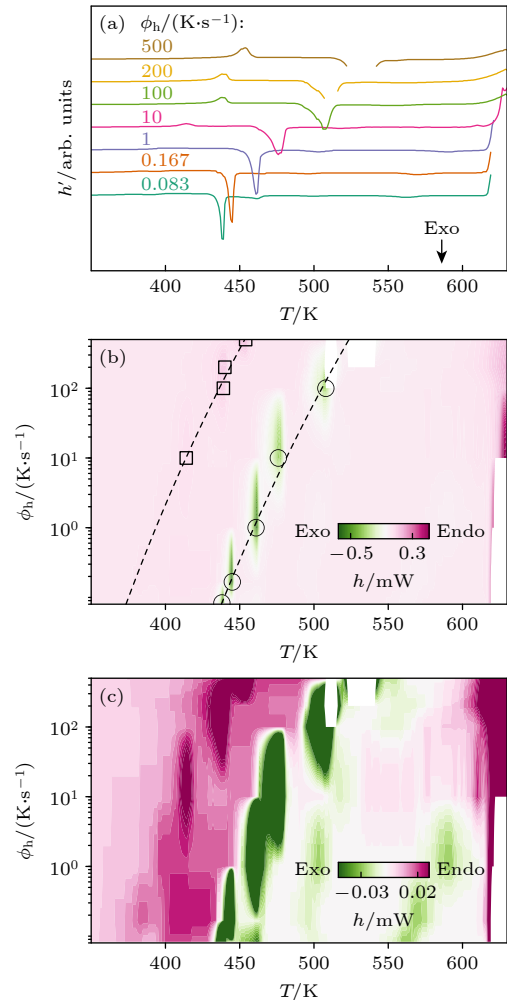
图 3 铸态 Au 基非晶合金的超快加热曲线 (a) 侧视图; (b) 俯视图; (c) 低热流强度下的俯视图. 方块和圆圈分别代表焓过冲和晶化的峰值温度; 信息数据来源于文献 [22]. 注: 由于文献 [22] 未能提供部分曲线上完整的晶化峰或熔化峰信息, 所以部分热流曲线不连续
