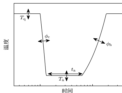
图 1 FDSC 实验的温控程序 ( T_q 代表熔体温度, T_a 代表退火温度, \phi_c 代表冷却速率, \phi_h 代表加热速率, t_a 代表退火时间; 双箭头代表变量可以调节的方向)
