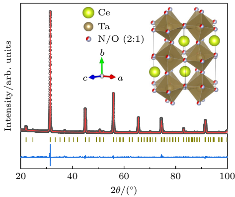
图 2 室温下 CeTaN 2 O 的 XRD 图谱和结构精修结果, 插图给出了晶体结构示意图
