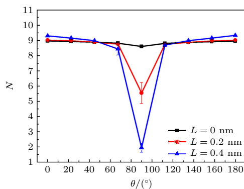
图 3 完整纳米通道及断裂纳米通道内的水分子平均占据数 ( N ) 随 \theta 的变化
