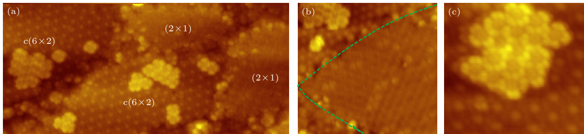
图 6 (a) 在 \text{Cu}_5\text{O}_6\text{-c}(6\times 2) 表面上沉积约 0.2 MLE 铈原子并吸附约 1.1 MLE VOPc 分子后获得的 STM 形貌图 ( 47\text{ nm}\times 22\text{ nm} , U=2.0\text{ V} , I=0.2\text{ nA} ), 图中存在两种不同的组装结构; (b) 扫描区域缩小后获得的 STM 图像 ( 26\text{ nm}\times 24\text{ nm} , U=2.0\text{ V} , I=0.2\text{ nA} ), 两种不同的组装结构用绿色虚线分隔; (c) 在 \text{Cu}_5\text{O}_6 区域缩小扫描范围后获得的 STM 形貌图 ( 15.6\text{ nm}\times 15.6\text{ nm} , U=2.0\text{ V} , I=0.2\text{ nA} )
