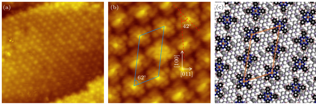
图 5 (a) 0.9 MLE VOPc 分子沉积在 \text{Cu}_5\text{O}_6\text{-c}(6\times 2) 表面后获得的 STM 形貌图 ( 24\text{ nm}\times 24\text{ nm} , U=2.5\text{ V} , I=0.2\text{ nA} ); (b) 当覆盖度约为一个单层时获得的具有亚分子分辨的 STM 图像 ( 6.4\text{ nm}\times 6.4\text{ nm} , U=0.5\text{ V} , I=0.2\text{ nA} ), 平行四边形单胞用蓝线表示, 相邻两分子取向的夹角约为 42^\circ ; (c) 图 (b) 对应的分子组装结构模型图, 结构单胞用橙色四边形表示
