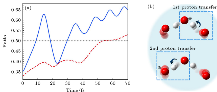
图 17 (a) 电离后轨迹 b (和图 16(b) 中的轨迹一致) 的从头算 Ehrenfest 动力学比图, 表示第一 (蓝色, 实线) 和第二 (红色, 虚线) 质子转移过程 [16] ; (b) 第一和第二质子转移示意图 [16]
