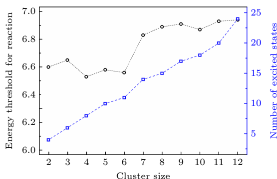
图 23 不同大小的水团簇中加入热电子的能量阈值 [40]
