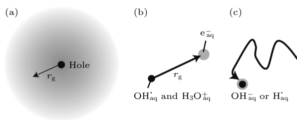
图11 过剩电子在水中的形成和定域过程示意图 (a) 辐射出的局部过剩电子 (灰色), 半径为 r_g [18] ; (b) 电子波函数的坍塌, 这将导致平均迁移长度为 r_g [18] ; (c) 扩散性成对重组 [18]
