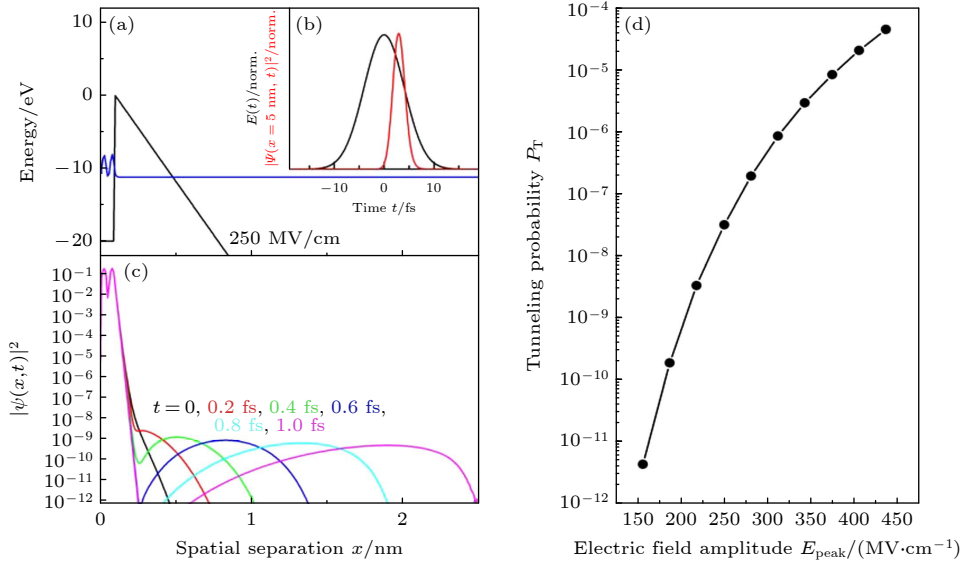
图 14 (a)–(c) 场诱导电子隧穿的分析 [19]; (d) 电子隧穿概率 P_T 与 10 fs 高斯驱动脉冲峰值电场的函数关系 (参见图 (b)) [19] Fig. 14. (a)–(c) Spatio-temporal aspects of field-induced electron tunneling [19]; (d) electron tunneling probability P_T as a function of the peak electric field of a 10-fs Gaussian driving pulse (cf. panel (b)) [19].
