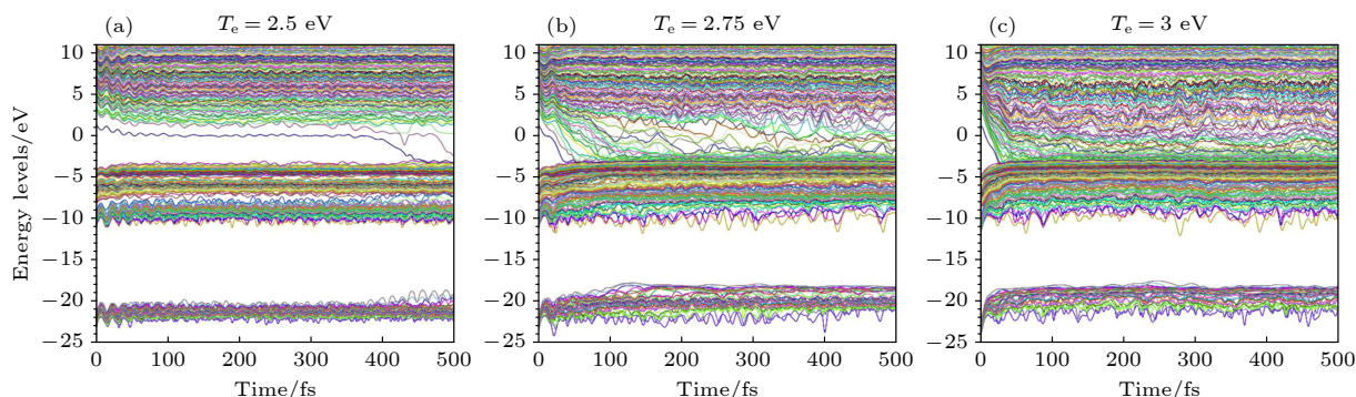
图 28 (a) 第一性原理计算得到的 1.6 eV/原子, (b) 2 eV/原子和 (c) 2.5 eV/原子情况下超快能量沉积中水的电子能级演化 [45]
