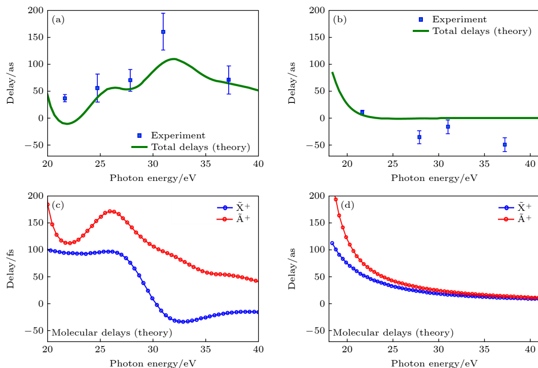
图 2 (a) 计算和测量得到的光电子从 \text{N}_2\text{O}^+ 的 \tilde{A}^+ 和 \tilde{X}^+ 态离开的时间延迟 [16]; (b) 与图 (a) 相同, 针对 \text{H}_2\text{O} 分子 [16]; (c), (d) 对于两个物种计算得到的分子延迟 [16]
