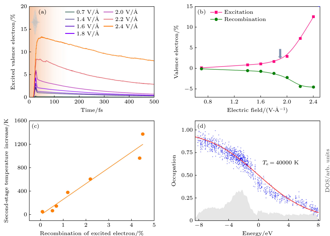
图 27 液态水电子动力学 (a) 受激价电子随激光脉冲电场的演化 [26] . (b) 激光脉冲电场下的有效电子激发和电子复合. 箭头显示了从多光子到强场电离过程的转变 [26] . (c) 电子复合与离子子系统第二阶段升温的关系 [26] . (d) 模拟中电场为 2.4 \text{ V/\AA} 时 t = 100 \text{ fs} 的电子占据, 给出了态的瞬时电子密度 [26] .
