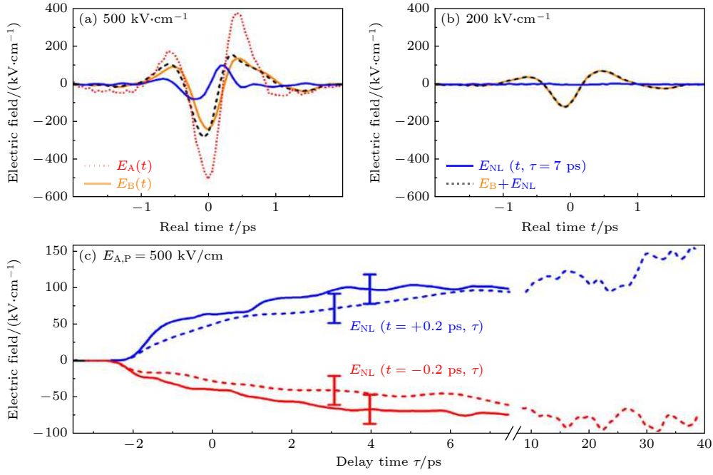
图 13 时间分辨非线性太赫兹响应 (a), (b) 延迟时间为 \tau = 7 \text{ ps} 时的非线性信号场 E_{NL}(t, \tau = 7 \text{ ps}) (蓝线)、探测场 E_B(t) (橙色线) 以及二者的和 E_{B,T}(t, \tau = 7 \text{ ps}) = E_B(t) + E_{NL}(t, \tau = 7 \text{ ps}) (黑色虚线) 都是入射脉冲 A 峰值振幅为 E_{A,P} = 500, 200 \text{ kV/cm} 时真实时间 t 的函数。场 E_{B,T}(t, \tau = 7 \text{ ps}) 代表通过激发样品传输的总 THz 探针场。图 (a) 中的红色虚线表示传输的泵浦场 E_A(t) [19]。 (c) 非线性信号场 E_{NL}(t = \pm 0.2 \text{ ps}, \tau) 作为在泵浦电场峰值振幅 E_{A,P} = 500 \text{ kV/cm} 下, t = -0.2 \text{ ps} (图 (a) 中的红色实线, 信号最小值) 和 t = +0.2 \text{ ps} (图 (a) 中的蓝色实线, 信号最大值) 时的延迟时间 \tau 的函数。虚线来自通过稍微改变泵浦场条件, 进行的符合实验精度范围 (误差条) 且有更长的延迟时间 \tau 的轨迹 [19]
