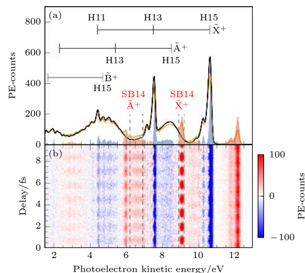
图 1 (a) H 2 O 分子的光电子能谱 [16] ; (b) IR-XUV 延迟的差谱 [16]
