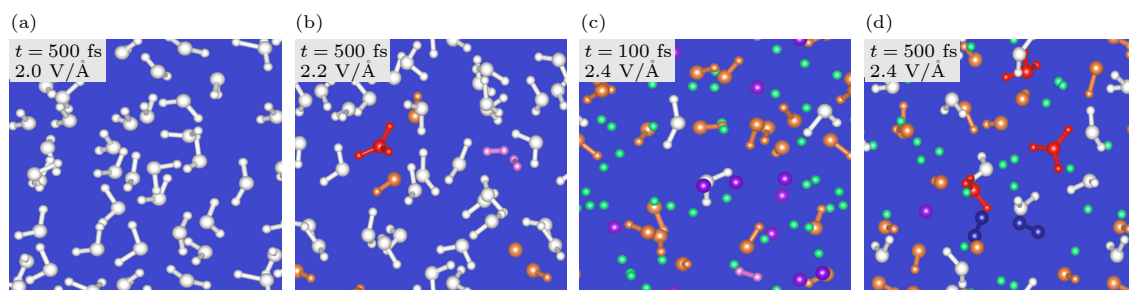
图 25 (a)–(d) 非绝热从头算分子动力学模拟构型. 激光脉冲的电场和时间如图所示. 水分子、水合离子、羟基、自由质子和氧原子、瞬态氢分子和氧分子分别显示为白色、红色、橙色、绿色、紫色、粉红色和深蓝色 [26]
