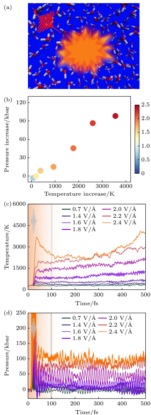
图 24 液态水的光致动力学 (a) 800 nm 激光脉冲照射液态水的示意图 [26] ; (b) 离子温度随体系压力的增加而增加, 色条表示脉冲的电场, 单位为 V/Å [26] ; (c) 离子温度随激光脉冲电场的时间演变, 光场包络线如插图所示, 这条竖线标志着第一阶段和第二阶段的分界 [26] ; (d) 液态水的两步离子加热 [26]
