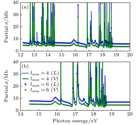
图 6 在两组不同角动量截断下用 XCHEM 计算获得的 \text{H}_2\text{O} 单光子电离的方向平均部分截面. 计算考虑了 12 至 19 eV 之间的能量区域 (a) 离开 \tilde{X}^2B_1 态离子的部分电离截面 [32] ; (b) 离开 \tilde{A}^2A_1 态离子的部分电离截面. 蓝色和绿色分别对应长度规范 ( L ) 和速度规范 ( V ). 实线和点线分别对应最大角量子数 l_{\max} 为 4 和 6 [32] .
