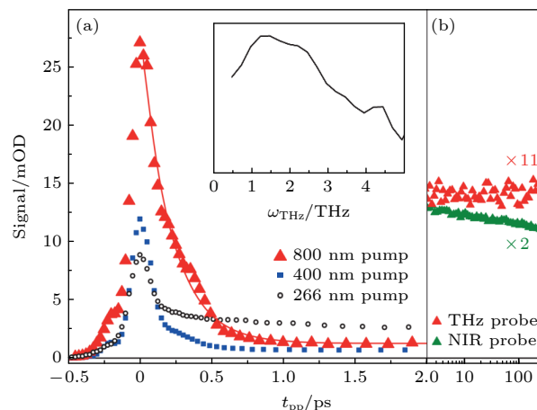
图10 纯水光电离的太赫兹响应 (a) 800 nm 泵浦 (红色三角形) 与单指数拟合结果 (200 fs, 红线)、400 nm 泵浦 (蓝色填充方形) 和 266 nm 泵浦 (黑色开口圆圈) 的结果. 400 和 266 nm 波长的泵浦轨迹以 800 nm 波长泵浦的水合电子 ( e_{aq}^- ) 浓度进行了缩放. 插图: 通过二维扫描推导出的 800 nm 泵浦时过量电子的光谱特征. 该初始光谱在约 1.5 THz 处达到峰值 [18] . (b) 使用 800 nm 泵浦 (红色, 按 11 倍缩放) 的长时间太赫兹响应保持不变, 而在近红外条件下探测到的响应则清楚地显示了成对重组的动力学 [18]
