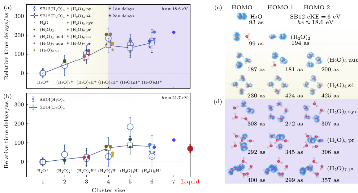
图3 水团簇的尺寸分辨光电离时间延迟 (a) 相对于 \text{H}_2\text{O} (或 \text{D}_2\text{O} ), 在 SB12 中测得的水团簇 1b_1 分波的光电离时间延迟 (空心圆圈). 误差条代表 95% 的置信区间. 计算的延迟 (实心符号) 是在 6.0 eV 的动能下得到的 [15] . (b) 与图 (a) 相同, 但对应于边带 SB14, 其中计算值是在 9.1 eV 的动能下得到的. 单光子 ( 1h\nu ) 和双光子 ( 2h\nu ) 延迟计算结果分别以实心圆圈和星形表示 [15] . (c), (d) 不同尺寸水团簇 1b_1 轨道 1—3 HOMO (记作 HOMO- i ) 的电子密度图和计算的光电离延迟. 在图 (c) 中以黄色背景表示了电子基本在整个团簇上离域, 而图 (d) 中紫色背景表示只定域在部分水分子上的情况 [15] .
