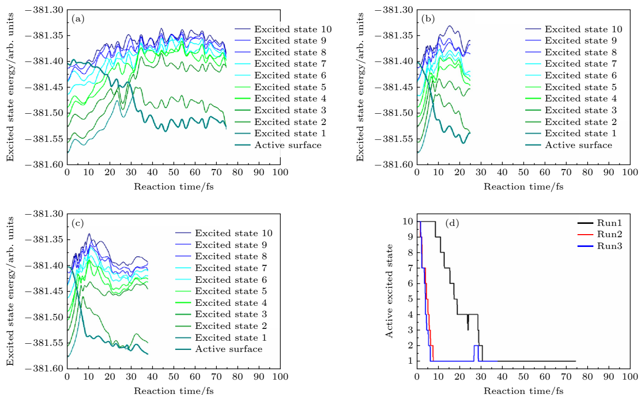
图 21 FSSH 的激发态表面和活性表面分别为第 1–3 次轨迹 (分别对应 (a)–(c)), 作为时间的函数, 对于五个水分子簇和一个初始激发态被选为第 10 激发态的电子. 青色粗曲线表示 FSSH 计算中任何时刻的“活化”状态. D1, D2 和更高级能级之间的能量分离表明电子在 OH 上的状态与电子在 H 上的状态 (对于相同的结构) 是相关的 [40] . (d) 活性激发态表面轮廓随反应时间的变化 [40]
