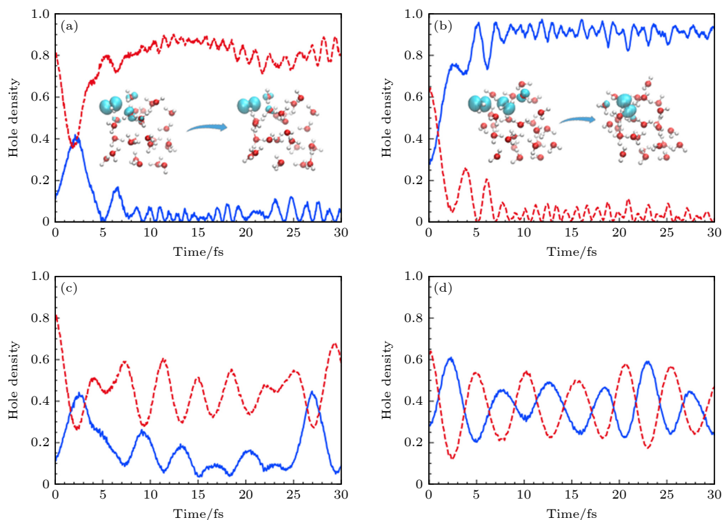
图 16 (a), (b) 采用从头算 Ehrenfest 动力学的选择模拟的时间分辨空穴密度图 [16] ; (c), (d) 固定核实时电子动力学, 初始条件分别与子图 (a) 和图 (b) 相同. 空穴密度是用在氧原子上的 Mulliken 自旋密度来计算的, 绘制的是两个最大的空穴密度 [16]
