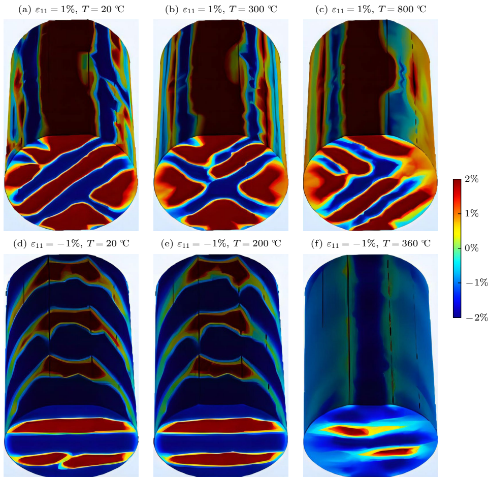
图 5 不同表面应力下 PTO 纳米线随温度变化的 \epsilon_{11} 分布 (a)—(c) \epsilon_{11} = 1\% ; (d)—(f) \epsilon_{11} = -1\%
