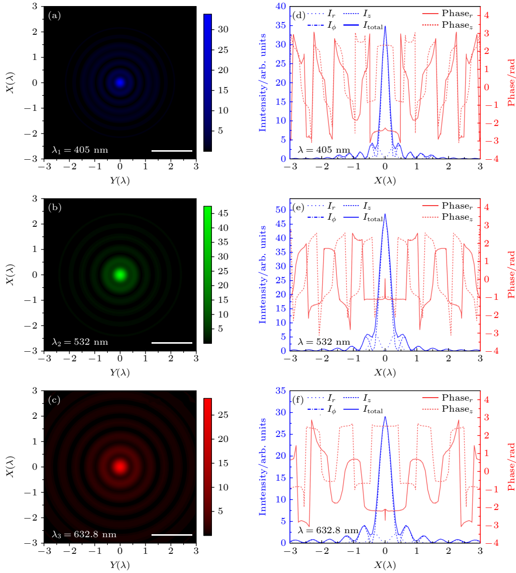
图 7 (a)–(c) \lambda_1 = 405 nm, \lambda_2 = 532 nm 和 \lambda_3 = 632.8 nm 入射条件下焦平面上的光场强度分布仿真结果; (d)–(f) 沿半径方向上不同分量的光场强度分布和相位分布
