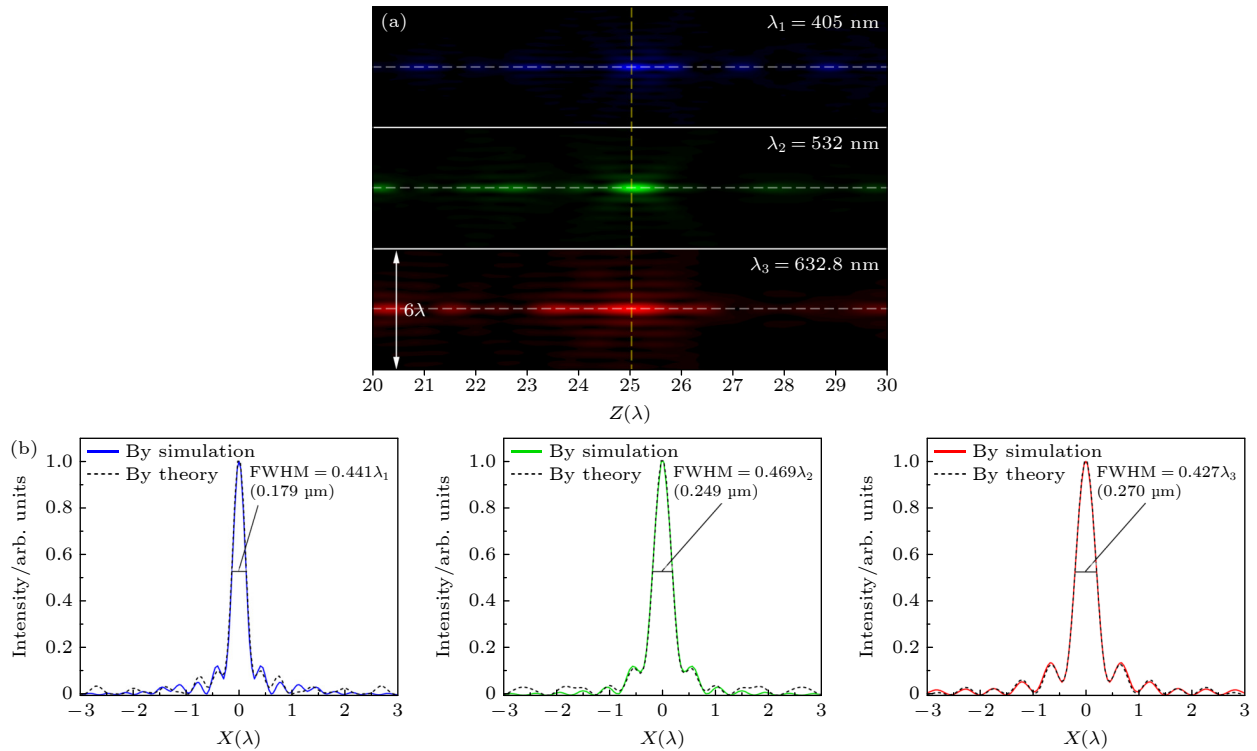
图 6 (a) \lambda_1 = 405 nm, \lambda_2 = 532 nm 和 \lambda_3 = 632.8 nm 入射条件下传播平面上和焦平面上的归一化光场强度分布仿真结果; (b) 通过焦斑中心沿半径方向上的光场强度分布
