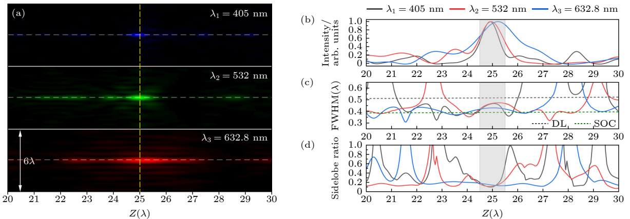
图5 (a) \lambda_1 = 405 nm, \lambda_2 = 532 nm 和 \lambda_3 = 632.8 nm 入射条件下传播平面上的光场强度分布; (b)–(d) 沿传播方向上峰值强度、半高全宽和旁瓣比率分布
