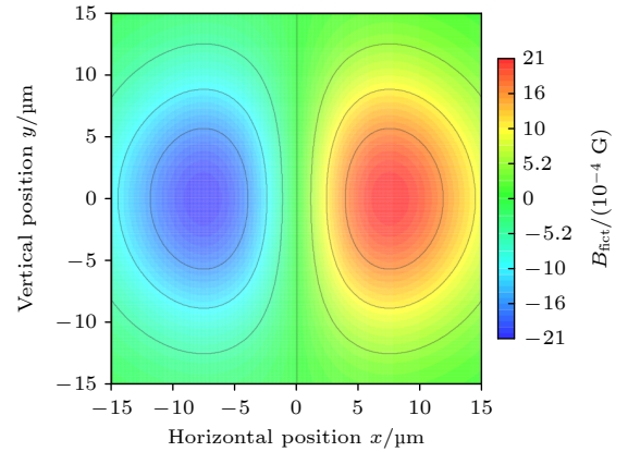
图 A1 聚焦偶极阱阱深最大 ( Z = 0 ) 处横截面的虚磁场梯度图. 偶极阱激光传播方向为 Z , 偏振方向为 X
