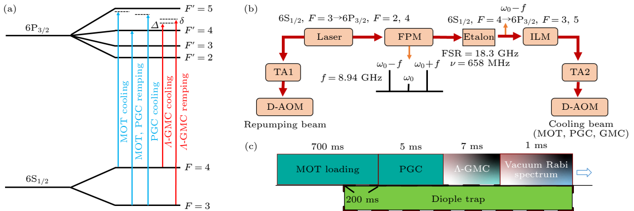
图 1 (a) 铯原子 D2 线能级图; (b) 快速、宽范围调谐激光系统产生过程, TA 为锥形放大器, Laser 为激光器, FPM 为光纤位调制器, Etalon 为标准具, ILM 为注入锁定放大, D-AOM 为双通声光调制器; (c) 时序图
