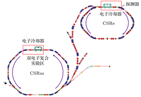
图 2 储存环 CSR m 与 CSR e 上的双电子复合实验平台示意图
