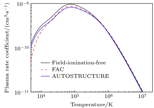
图 8 Kr 25+ 离子的实验(黑色实线)与FAC(红色虚线)及AUTOSTRUCTURE [22] (蓝色实线)理论导出的等离子速率系数谱对比
