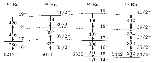
图7 ^{130}\text{Ba} [37], ^{131}\text{Ba} , ^{132}\text{Ba} [49]和 ^{133}\text{Ba} [59]中 \Delta I=1 跃迁序列的能级间隔系统性
