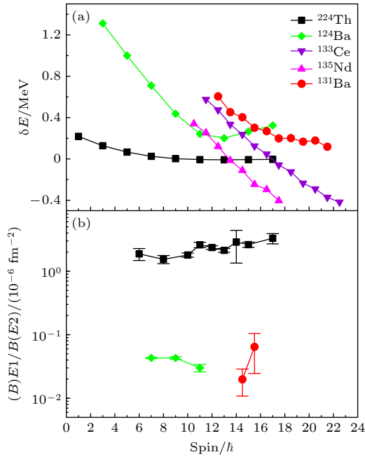
图 5 ^{131}\text{Ba} , ^{124}\text{Ba} [24], ^{224}\text{Th} [38], ^{133}\text{Ce} [39] 和 ^{135}\text{Nd} [36] 中 (a) 能量移动 \delta E 和 (b) 正负宇称带间的约化跃迁分支比 B(E1)/B(E2) 随自旋变化
