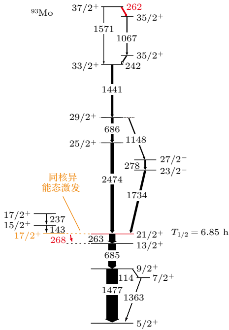
图 3 ^{93m}\text{Mo} 能级纲图
