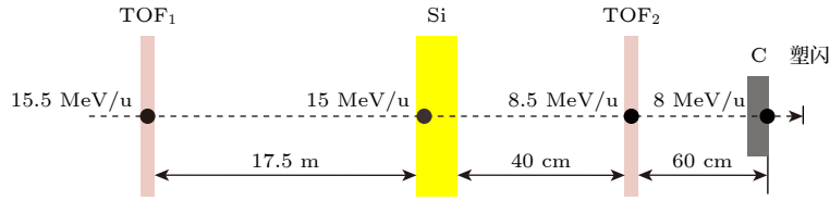
图 5 实验设置示意图
