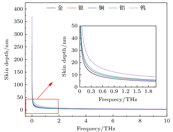
图 1 五种常见金属在太赫兹波段的趋肤深度随频率的变化关系
