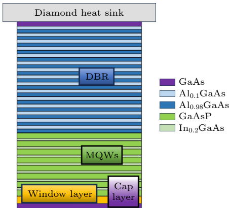
图 1 增益芯片外延结构简图
