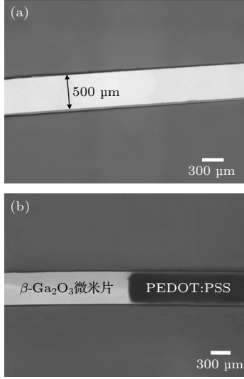
图 2 (a) 单根 \beta -Ga 2 O 3 微米片的 SEM 图; (b) 单根 PEDOT:PSS/ \beta -Ga 2 O 3 异质结的 SEM 图
