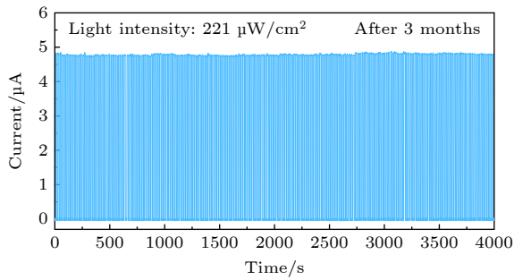
图 7 3 个月, 器件在 0 V 偏压下的时间响应
