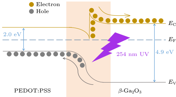
图 8 PEDOT:PSS/ \beta\text{-Ga}_2\text{O}_3 异质结光电器件在 254 nm 和 0 V 偏压下的能带图
