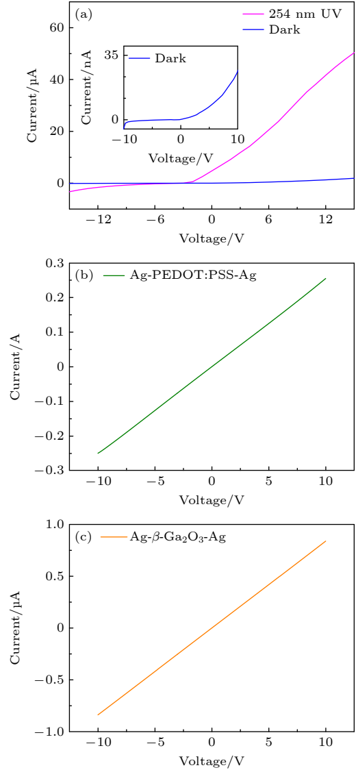
图 3 (a) 器件在黑暗和 254 nm 光照下的 I - V 曲线, 插图为黑暗条件下器件的 I - V 曲线; (b) Ag-PEDOT:PSS-Ag 的 I - V 曲线; (c) Ag- \beta -Ga 2 O 3 -Ag 的 I - V 曲线
