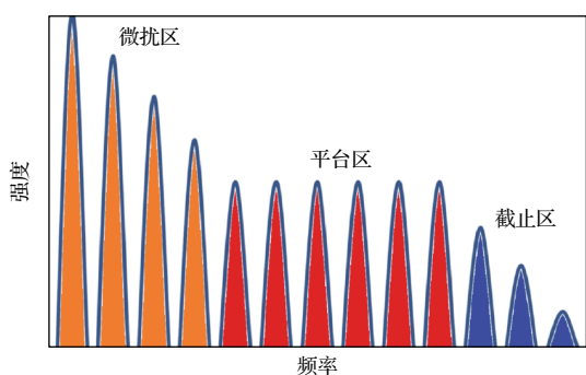
图 11 高次谐波的典型特征
