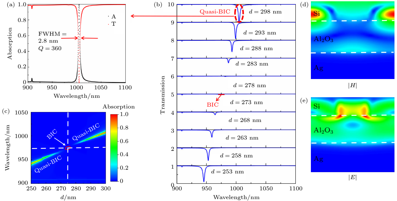
图 3 (a) Si/Al 2 O 3 /Ag 超材料吸收器的吸收光谱和透射光谱; (b) 参数 d 变化对吸收光谱的影响; (c) BIC 和 q-BIC 与参数 d 的关系; (d) BIC 的磁场分布; (e) BIC 的电场分布
