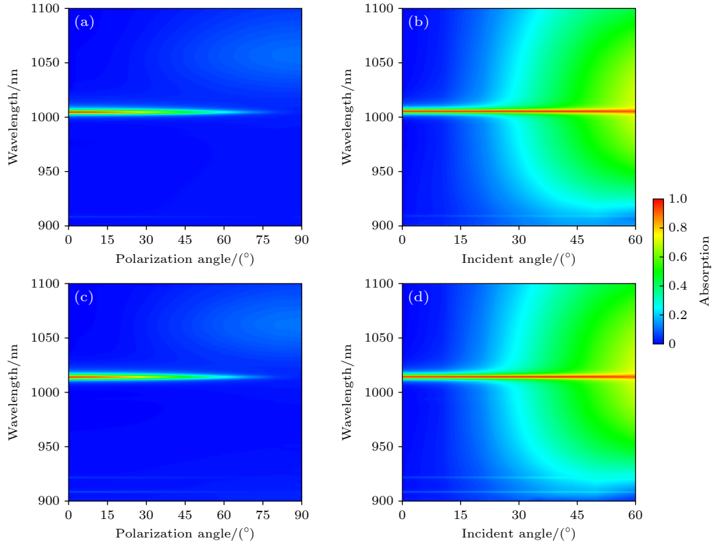
图 9 w = 155 nm 时, (a) 光源偏振角 \alpha 和 (b) 光源入射角 \theta 对 BIC 的影响; 分别是 w = 140 nm 时, (c) 光源偏振角 \alpha 和 (d) 光源入射角 \theta 对 BIC 的影响
