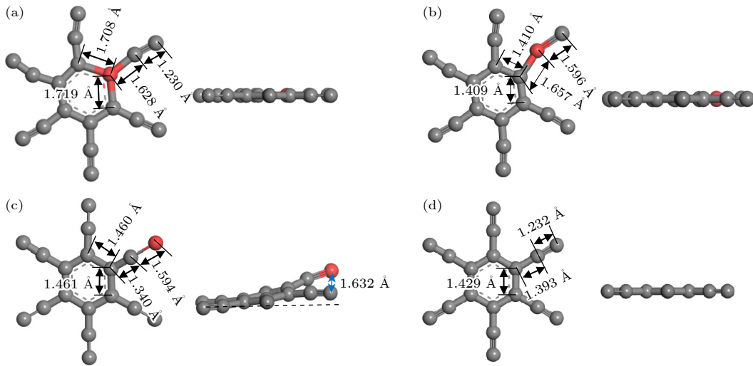
图 2 掺杂位与邻近碳原子之间的键长 (a) C_I 位; (b) C_{II} 位; (c) C_{III} 位; (d) 本征石墨炔
