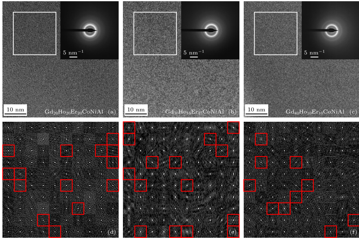
图 2 \text{Gd}_{20+2x}\text{Ho}_{20-x}\text{Er}_{20-x}\text{CoNiAl} ( x = 0, 5, 10 ) 非晶合金条带 HRTEM 图 (a)–(c) 及选区二维自相关处理图 (d)–(f), 插图选区电子衍射图
