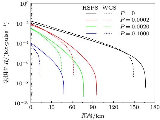
图 2 不同干涉误差下基于监控 HSPS 协议和基于监控 WCS 协议的密钥率对比
