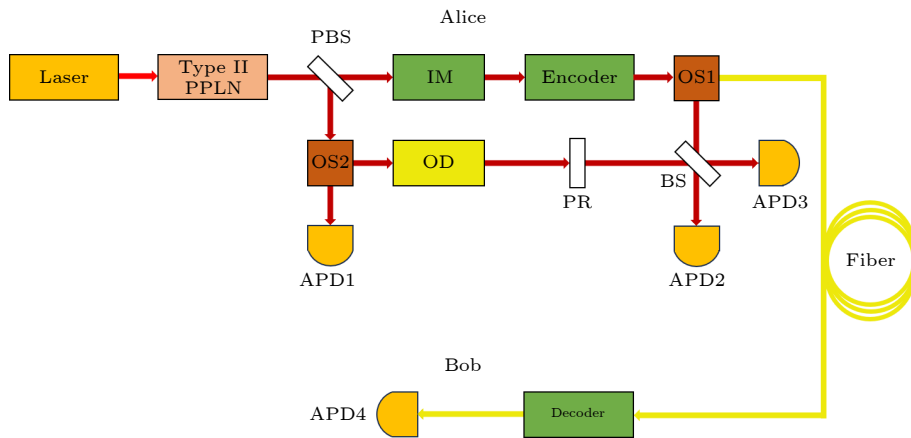
图 1 基于监控标记单光子源的 QKD 实验装置结构示意图
