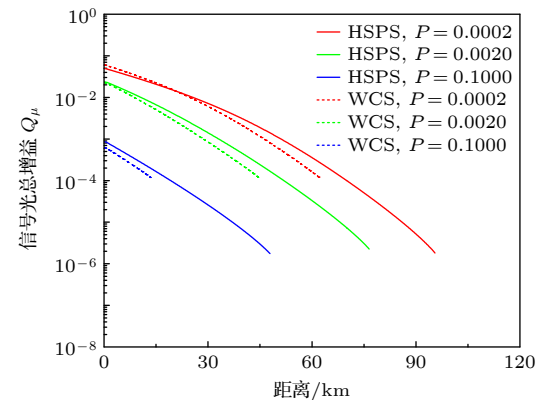
图 4 不同干涉误差下基于监控 HSPS 协议和基于监控 WCS 协议的信号光平均增益对比
