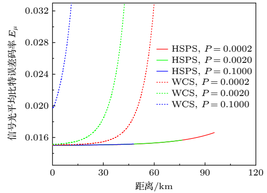
图 3 不同干涉误差下基于监控 HSPS 协议和基于监控 WCS 协议的平均误码率对比
