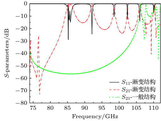
图 3 渐变结构的 S 参数 Fig. 3. The S-parameter of the gradient structure.
