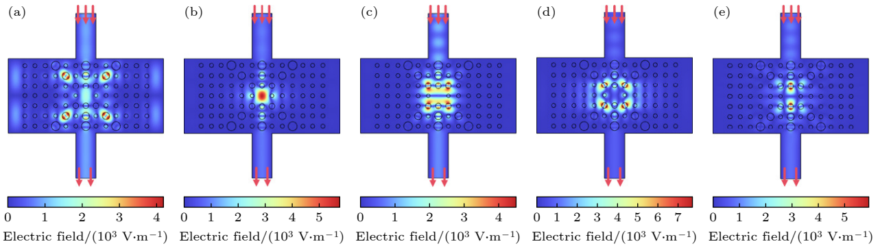
图 4 入射功率为 1 W 时渐变结构中的电场分布 (a) 85.2 GHz; (b) 92.1 GHz; (c) 98.5 GHz; (d) 102.4 GHz; (e) 106 GHz Fig. 4. Electric field distribution in gradient structure with incident power of 1 W: (a) 85.2 GHz; (b) 92.1 GHz; (c) 98.5 GHz; (d) 102.4 GHz; (e) 106 GHz.
