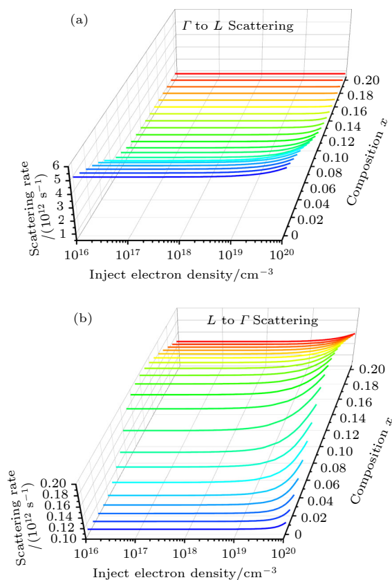
图 3 谷间散射率与注入电子之间的关系 (a) \Gamma 能谷到 L 能谷的谷间散射率; (b) L 能谷到 \Gamma 能谷的散射率
