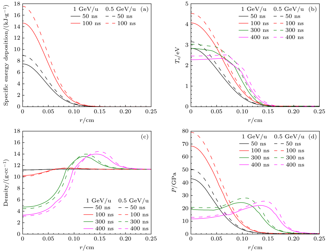
图 3 不同束团能量下, 束团强度为 1 \times 10^{11} ppp, 长度为 100 ns 的物态参数随半径的变化规律 (a) 离子束单位质量的能量沉积; (b) 电子温度; (c) 密度; (d) 压强
