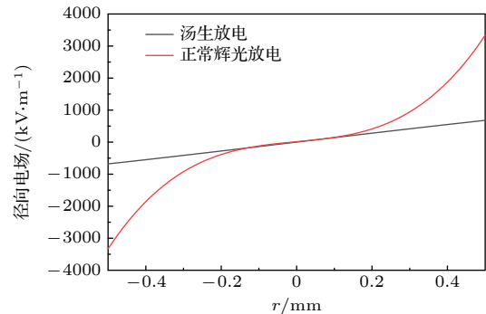
图 7 稳态放电模式下 z = -2.5 \text{ mm} 处一维径向电场
