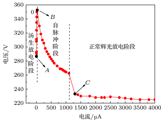
图 2 伏安特性曲线图
