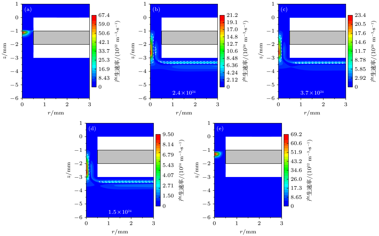
图 13 不同时刻电子产生速率分布图 (a) 58.9 μs; (b) 118.1 μs; (c) 131.3 μs; (d) 132.1 μs; (e) 146.3 μs
