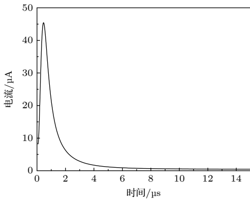
图 12 极间电压 270 V 时放电电流随时间变化图
