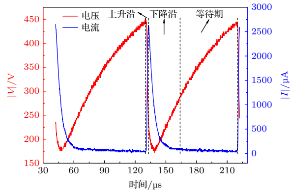
图 4 平均电流 250 \mu\text{A} 时的电压和电流脉冲波形图
