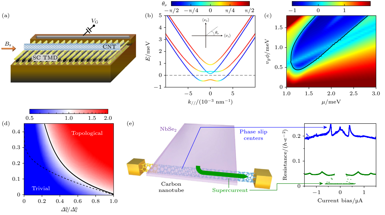
图6 碳纳米管-TMD 超导体异质结的拓扑态构建方案 (a) 碳纳米管-TMD 超导体异质结器件示意图, 在轴向磁场和横向电场下诱导出马约拉纳束缚态 [119] ; (b) 自旋轨道耦合、磁通效应、横向电场和伊辛近邻效应导致的半金属态碳纳米管; (c) 磁通和化学势的拓扑相图, -1 表示拓扑相 [119] ; (d) 电子-电子相互作用诱导的无磁场拓扑相图 [119] ; (e) 碳纳米管-薄层 NbSe 2 近邻下的超导电流和相滑移 [105]
