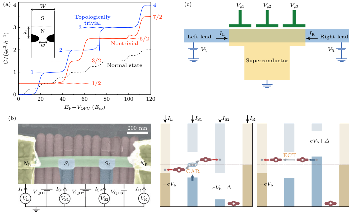
图3 拓扑态的固态量子器件构筑和探测 (a) 基于强自旋轨道耦合的二维电子气构筑超导界面和量子点接触的复合结构器件, 在磁场驱动下在拓扑相区域, 电导出现半整数的量子化平台 [72] ; (b) 三端非局域测量方案的器件构型, 用于区分安德列也夫和马约拉纳束缚态 [73] ; (c) 基于半导体纳米线与超导电极构筑耦合量子点的 Kitaev 链器件结构 [82] , 实验通过栅极实现对交叉安德列也夫反射和弹性共隧穿过程的精确调控 [81]
