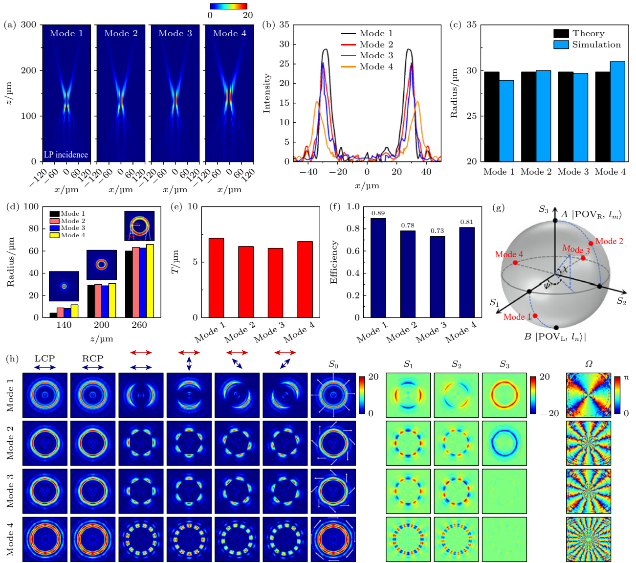
图 3 在 x -LP 光照射下, (a) 4 种模式 PVVBs 在 x - z 平面上电场强度分布; (b) 在焦平面上电场强度分布曲线; (c) 在焦平面上亮环半径; (d) 在 z = 140, 200 和 260 \mu\text{m} 三个横截面上的亮环半径; (e) 在焦平面上的亮环宽度; (f) 转化效率; (g) 在 HyOPS 上位置分布; (h) x -LP 光照射下, 4 种模式 PVVBs 在不同偏振片下对应的电场强度分布, 斯托克斯参数 ( S_0, S_1, S_2 和 S_3 ) 及偏振方向 ( \Omega ) Fig. 3. Under x -LP illumination, (a) the electric field intensity distributions of the four mode PVVBs in the x - z plane; (b) the intensity profiles at the focal plane; (c) the radii of the bright rings at the focal plane; (d) the radii of the bright rings at z = 140, 200 and 260 \mu\text{m} cross-sections; (e) the widths of the bright rings at the focal plane; (f) conversion efficiency; (g) their spatial distributions on the HyOPS; (h) under x -LP illumination, the electric field intensity distributions, Stokes parameters ( S_0, S_1, S_2 and S_3 ) and polarization orientations ( \Omega ) of the four mode PVVBs under different polarizers.
