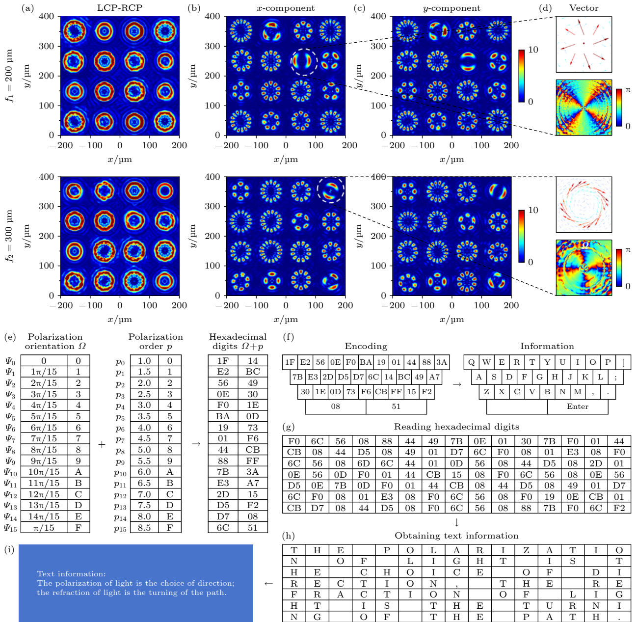
图 4 超构表面 MF5 在 LCP 光下生成 RCP PVBs 阵列的电场强度分布图 (a) 及在 LP 光下生成的 32 重 PVVBs E_x 分布图 (b) 和 E_y 分布图 (c); (d) 对应模式 PVVBs 的矢量场分布和偏振角度分布; (e) PVVBs 代码表; (f) 编码方法和编码表; (g) 105 个包含两字节的十六进制数字序列; (h), (i) 解密的文本信息
