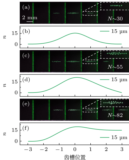
图 2 尘埃等离子体金属直棘轮中尘埃颗粒的正流 (a), (c), (e) 随着投入尘埃颗粒数的增加, 尘埃颗粒在棘轮通道中的空间分布逐渐向右扩展, 形成正向整流, 图中 N 代表棘轮通道中尘埃颗粒总数量; (b), (d), (f) 对应的不同锯齿槽位置处颗粒数 n 的分布情况, 放电气压 p = 35 Pa, 放电功率为 P = 40 W, 颗粒直径为 15 \mu\text{m} . 图中尘埃颗粒做了亮度增强处理
