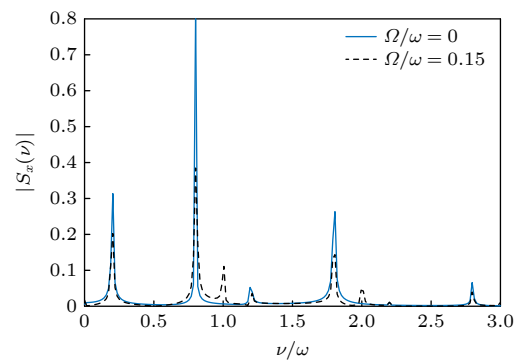
图 6 \Omega = 0 (蓝色实线) 和 \Omega = 0.15\omega (黑色虚线) 时自旋频谱 |S_x(\nu)| 的取值, 驱动参数固定为 \zeta = 100\sqrt{\hbar/(\pi m\omega)} , \eta = 0 , 其他参数以及初态选择与图 3 一致
