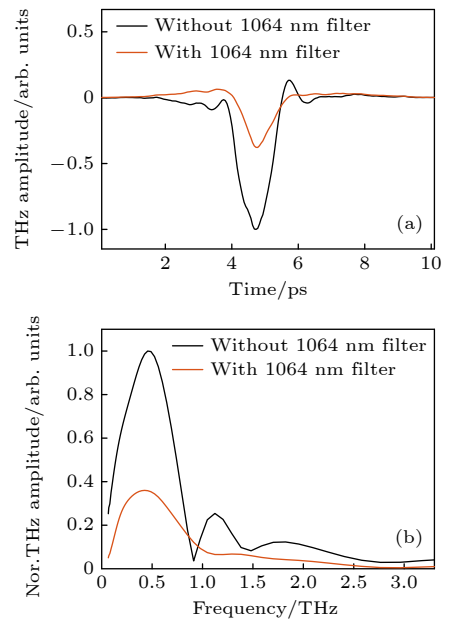
图 7 1064 nm 成分泵浦电光晶体产生 THz 辐射
