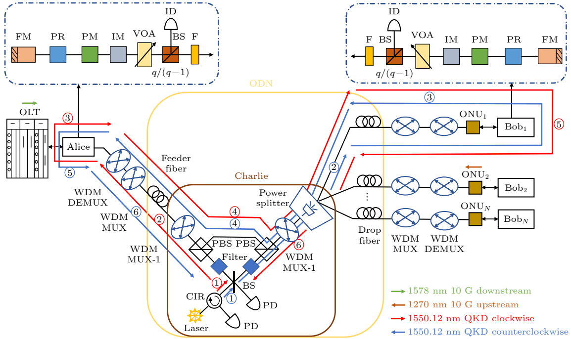
图 9 即插即用双场量子接入网络与 10 G-以太网无源光网络的全共存架构 [56]
