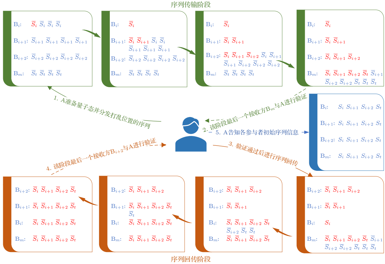
图 3 有新的接收方加入时的协议流程, 其中红色标注的量子序列是在传输阶段参与者进行保留的序列, 蓝色标注的量子序列是在传输阶段不同参与者的传输回合中待发送的序列
