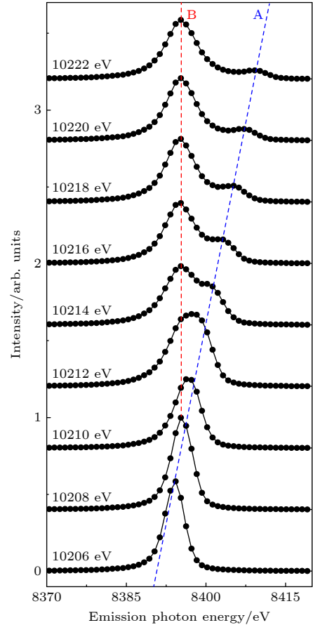
图5 WSi_2 在 10206—10222 eV 入射光能量激发下的荧光谱, 对应图 4(a) 垂直剖面. 其中蓝色虚线对应 2p-5d 共振荧光峰 (A 峰); 红色虚线对应 8397.6 eV 的 W- L\alpha_1 非共振荧光峰 (B 峰)
