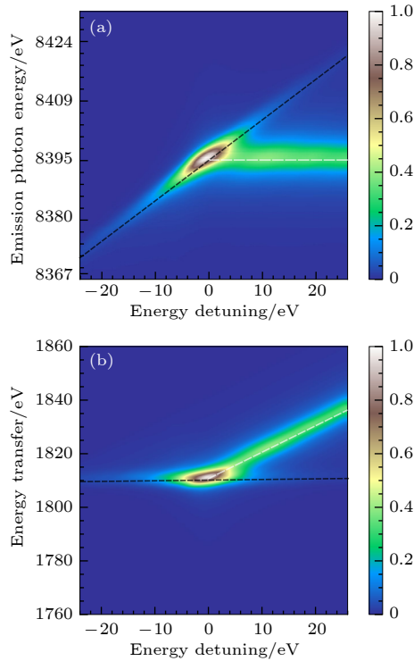
图4 W 的 L_3 吸收边 (10208 eV) 附近的 RIXS 二维图 (a) 及能量转移图 (b). 白色虚线对应发射光能量为 8397.6 eV, 对应 2p 电子电离产生 2p^{-1}\epsilon d 中间态过程. 此时随入射光能量的增加发射光子能量不变, 能量转移变大. 黑色虚线对应能量转移约为 1809 eV, 对应 2p-5d 共振产生 2p^{-1}5d 中间态过程. 此时随入射光能量的增加, 发射光子能量增加但能量转移保持不变
