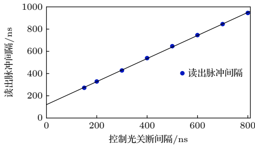
图 3 入射脉冲与控制光的时间间隔和读出脉冲间隔的关系曲线
