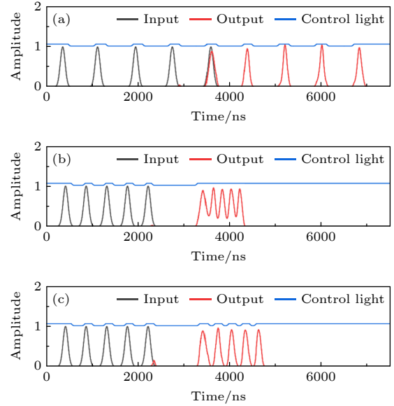
图 4 五脉冲存储读取图
