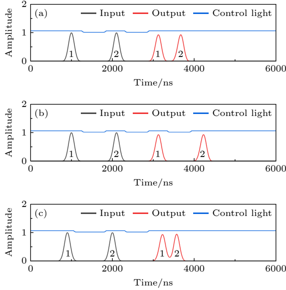
图 2 随机时间间隔两脉冲 EIT 存储读取示意图, 黑色为入射脉冲, 红色为读出脉冲, 蓝色代表控制光关断情况, 高电平为打开, 低电平为关断
