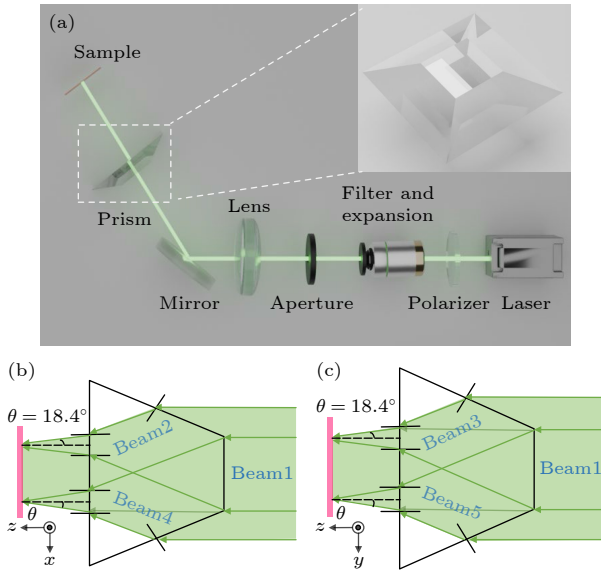
图 9 五波干涉光路制备光栅 (a) 整体光路图; (b) 棱台分光 x - z 平面示意图; (c) 棱台分光 y - z 平面示意图
