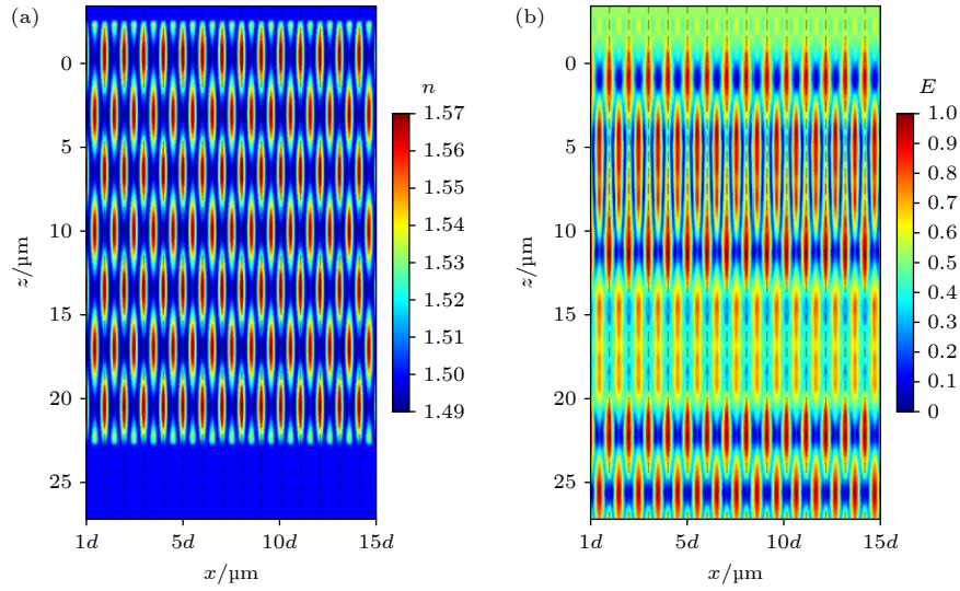
图 4 光栅厚度 25\ \mu\text{m} 、曝光光强比 1.0 条件下一维光栅仿真 (a) 光栅折射率分布图; (b) 衍射再现归一化电场图
