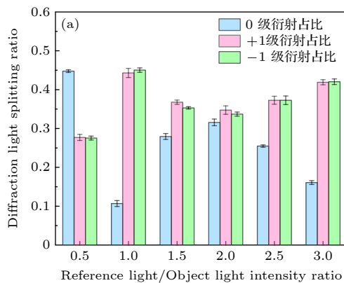
图 8 一维光栅实验结果 (a) 一维光栅样品测试数据; (b) 曝光光强比为 1.0 条件时分光图
