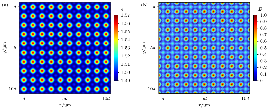
图 6 光栅厚度 25\text{ }\mu\text{m} 、曝光光强比 1.5 条件下二维光栅仿真 (a) 光栅折射率分布图; (b) 衍射再现归一化电场图
