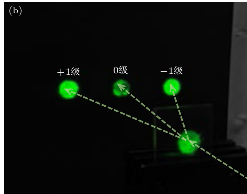
图 8 一维光栅实验结果 (a) 一维光栅样品测试数据; (b) 曝光光强比为 1.0 条件时分光图
