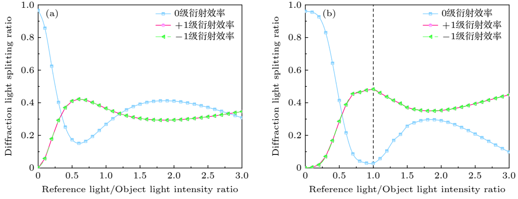
图 3 三波干涉一维光栅衍射分光占比随参考光/物光曝光光强比变化 (a) 厚度 10\ \mu\text{m} ; (b) 厚度 25\ \mu\text{m}
