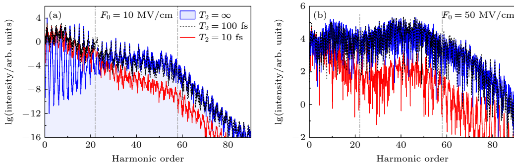
图 3 退相干时间 T_2 对一维 Fermi-Hubbard 模型高次谐波产生的影响 (a) 弱场驱动 ( F_0 = 10 MV/cm) 下不同退相干强度的谐波谱对比: 无退相干 ( T_2 = \infty , 蓝色实线)、中等退相干 ( T_2 = 100 fs, 黑色实线)以及强退相干 ( T_2 = 10 fs, 红色实线); (b) 强场驱动 ( F_0 = 50 MV/cm) 下的对应结果
