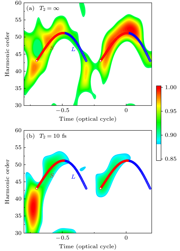
图 5 强场驱动 ( F_0 = 50 MV/cm) 下 30—60 阶高次谐波的时频分析 (Gabor 变换) (a) 无退相干情形 ( T_2 = \infty ), 时频谱中清晰分辨出对应半经典三步模型的短轨道 (红色曲线) 与长轨道 (蓝色曲线); (b) 引入强退相干 ( T_2 = 10 fs) 后, 长轨道 ( L ) 贡献显著抑制, 短轨道 ( S ) 信号保留并占据主导
