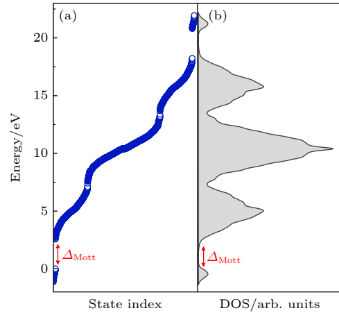
图 1 一维半填充 Fermi-Hubbard 模型的本征能级谱与态密度 (DOS) 的对应关系 (a) 采用精确对角化方法获得的本征能量分布 (蓝色散点), 横轴按态索引升序排列, 清晰显示有限尺寸效应导致的分立能级结构及强关联诱导的 Mott 能隙 \Delta_{\text{Mott}} ; (b) 对应的电子态密度分布 (黑色实线)
