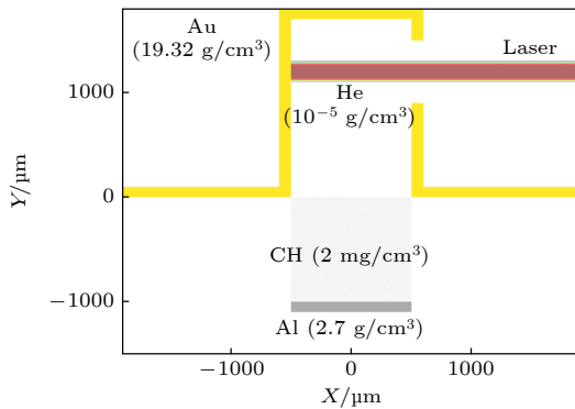
图 1 二维模型设置示意图 Fig. 1. Schematic of the 2D model setup.
