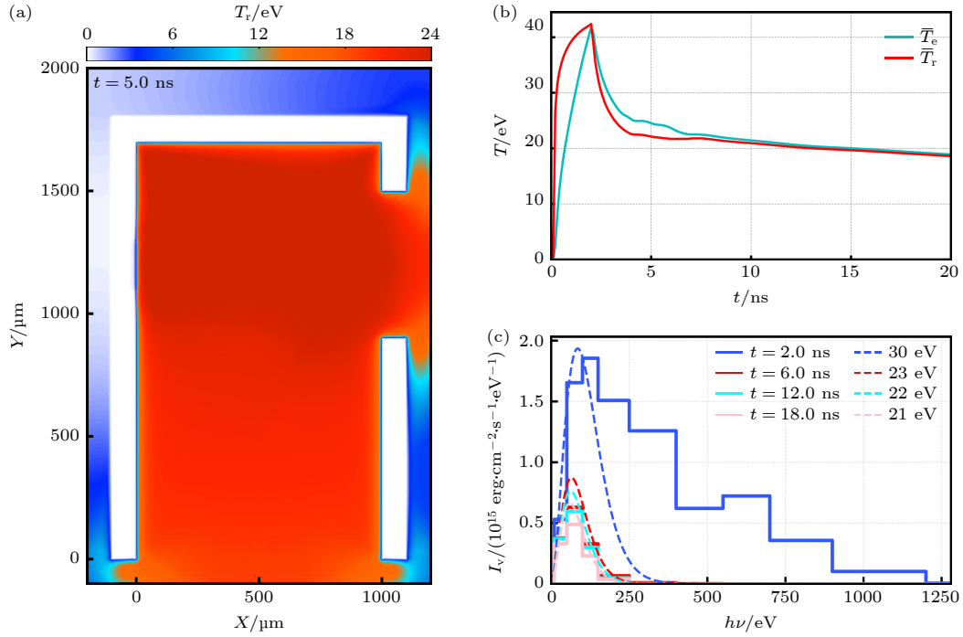
图 3 (a) t = 5.0 ns 时, 黑腔辐射温度 T_r 二维空间分布; (b) 黑腔平均电子温度 \bar{T}_e 与辐射温度 \bar{T}_r 演化; (c) 黑腔平均光谱强度 I_v 演化 (实线) 与对应的普朗克谱拟合曲线 (虚线)
