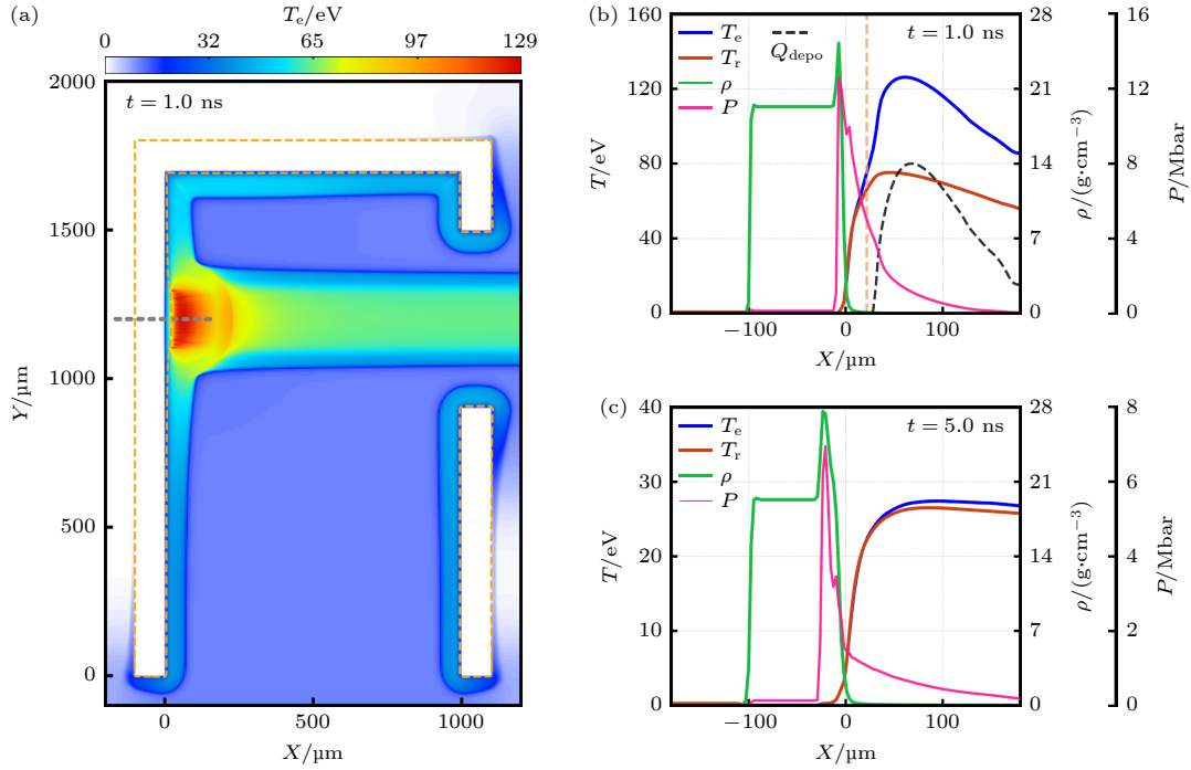
图 2 (a) t = 1.0 ns 时黑腔电子温度 T_e 的二维空间分布; (b), (c) t = 1.0 ns 和 t = 5.0 ns 时, Y = 1200 \mu\text{m} 处的电子温度 T_e 、辐射温度 T_r 、密度 \rho 和压强 P 的演化曲线. 图 (b) 中黄色虚线表示激光临界密度面, 黑色虚线表示归一化单位体积内的激光能量沉积密度
