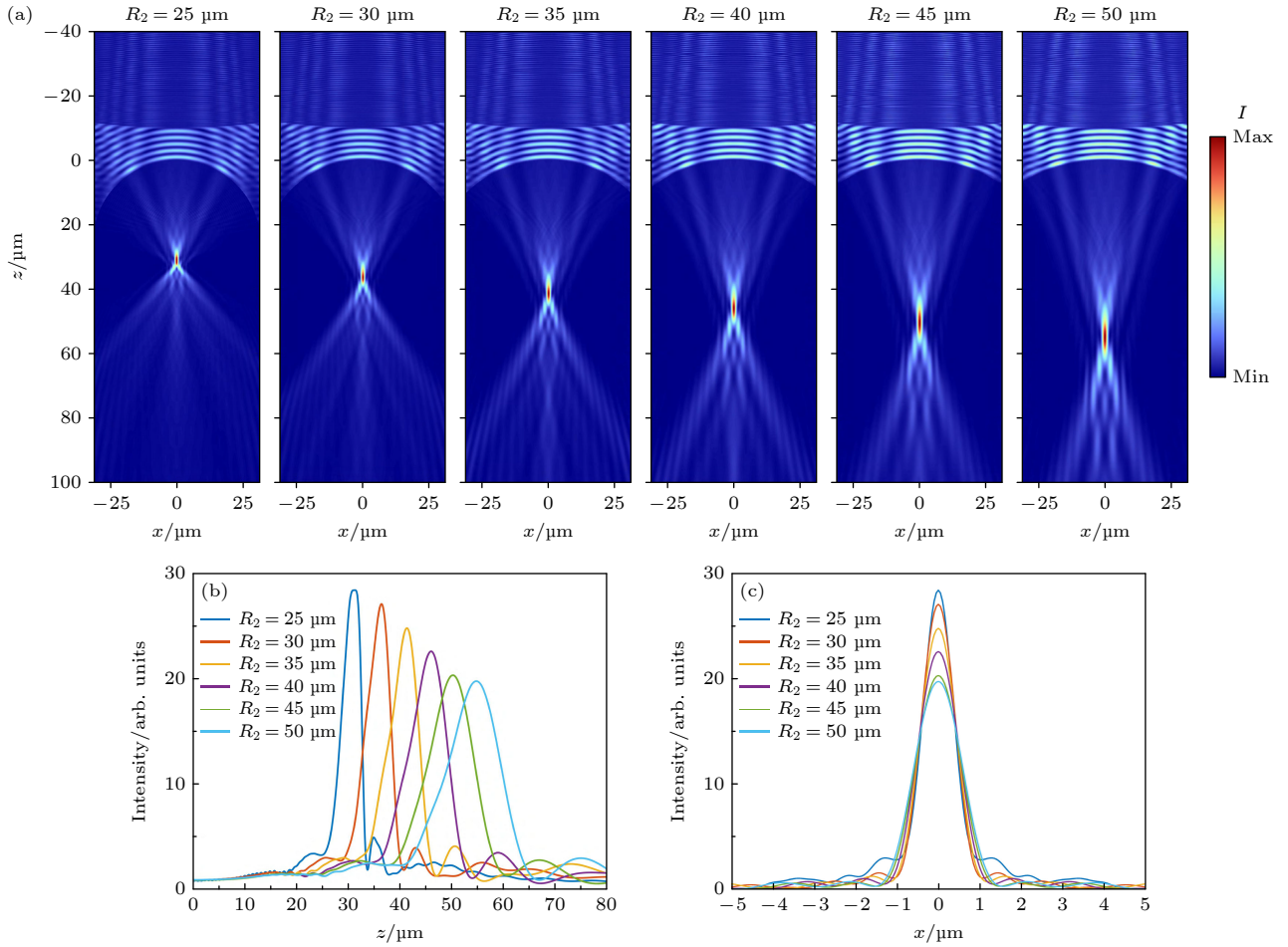
图4 对双凹型球面空气微透镜的前球面半径 R_2 的参数扫描仿真结果 (a) R_2 = 25 \mu\text{m} , 30 \mu\text{m} , 35 \mu\text{m} , 40 \mu\text{m} , 45 \mu\text{m} 和 50 \mu\text{m} 时, xOz 面的光强分布, 其中 R_1 的参数为 200 \mu\text{m} , t 为 10 \mu\text{m} ; (b) 沿传播方向 ( z 轴) 一维场强分布; (c) 焦点处的横向 ( x 轴) 一维场强分布
