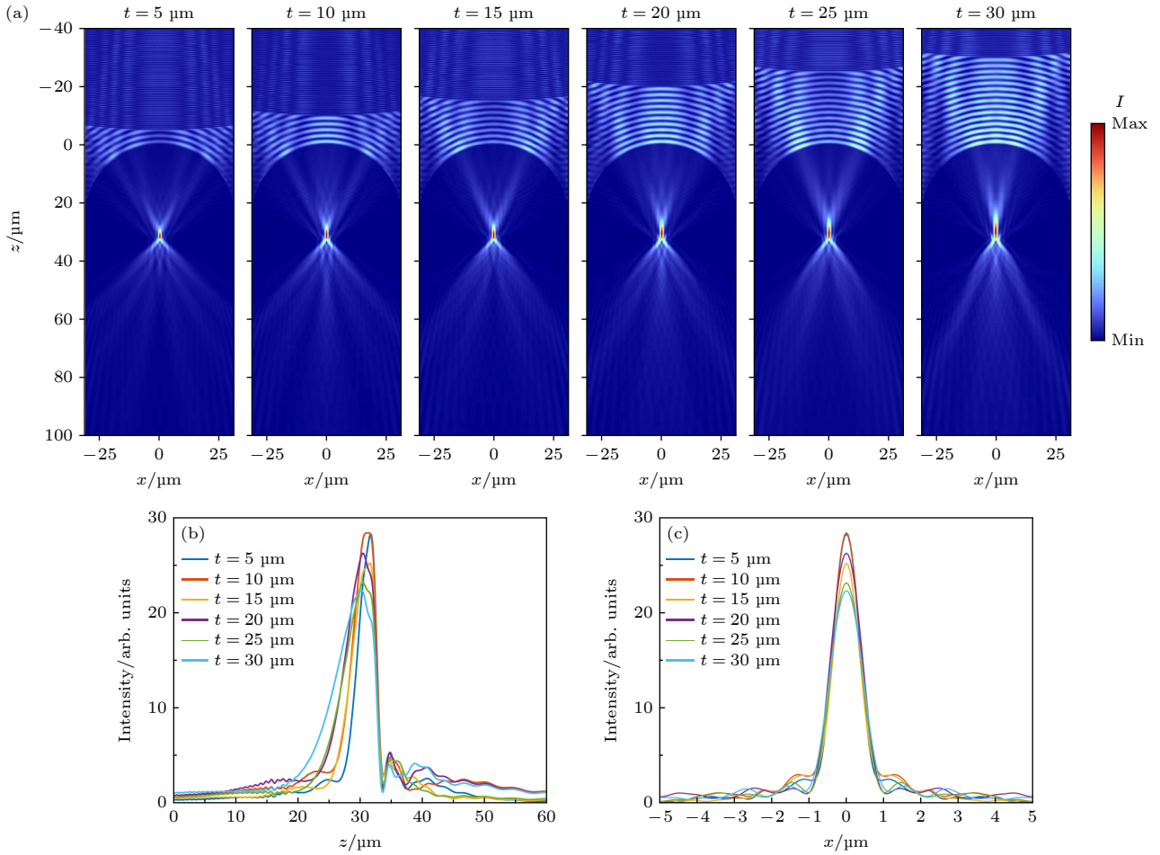
图 5 对双凹型球面空气微透镜的厚度 t 的参数扫描仿真结果 (a) t = 5, 10, 15, 20, 25 和 30 \mu\text{m} 时, xOz 面的光强分布; (b) 沿传播方向 ( z 轴) 一维场强分布; (c) 焦点处的横向 ( x 轴) 一维场强分布
