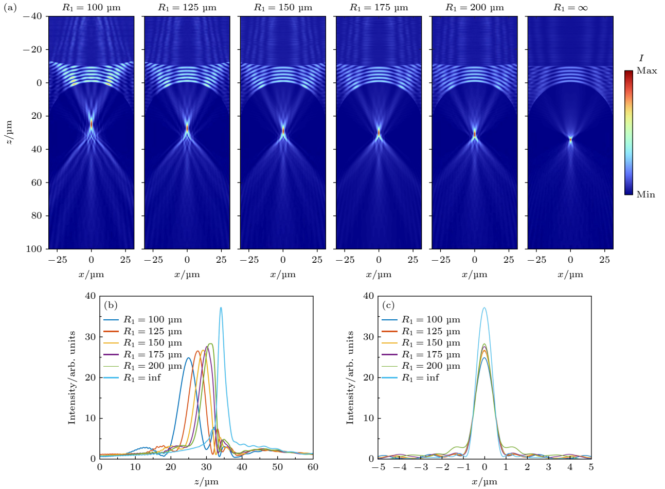
图 3 对双凹型球面空气微透镜的前球面半径 R_1 的参数扫描仿真结果 (a) R_1 = 100 \mu\text{m} , 125 \mu\text{m} , 150 \mu\text{m} , 175 \mu\text{m} , 200 \mu\text{m} 和 R_1 为平面结构时, xOz 面的光强分布, 其中 R_2 的参数为 25 \mu\text{m} , t 为 20 \mu\text{m} ; (b) 沿传播方向 ( z 轴) 一维场强分布; (c) 焦点处的横向 ( x 轴) 一维场强分布
