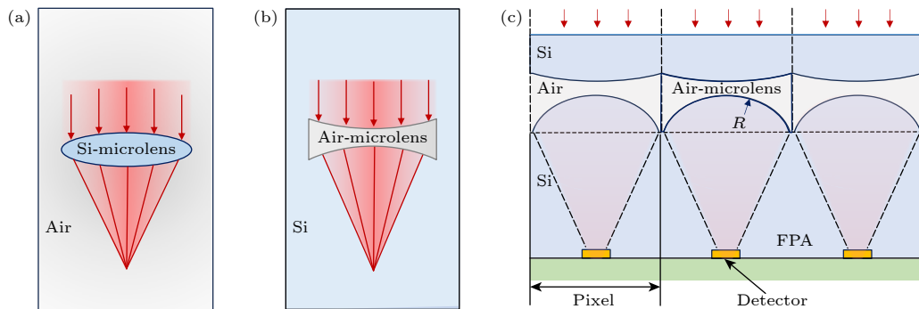
图 1 传统微透镜与空气微透镜设计对比 (a) 传统高折射率微透镜示意图; (b) 双凹型空气微透镜示意图; (c) 双凹型空气微透镜阵列集成于背照射红外焦平面阵列的二维剖面示意图, 展示了其在硅基底内部将入射光束高效汇聚并精准投射至底部微缩光敏元 (红外吸收层) 的工作机理
