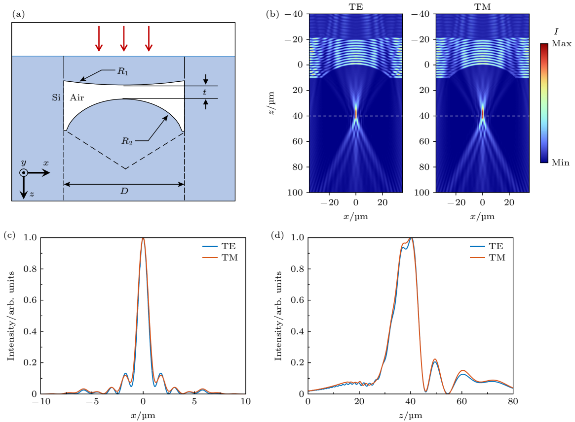
图 2 (a) 双凹型球面空气微透镜的剖面结构示意图, D , t , R_1 , R_2 分别为空气微透镜的直径、厚度、前表面半径和后表面半径; (b) TE 和 TM 偏振入射光下, 对参数为 t = 20\ \mu\text{m} , R_1 = 175\ \mu\text{m} , R_2 = 35\ \mu\text{m} 的双凹球面空气微透镜的聚焦场强仿真结果; (c), (d) 分别为沿焦点的 x 轴和 z 轴截面的场强分布
