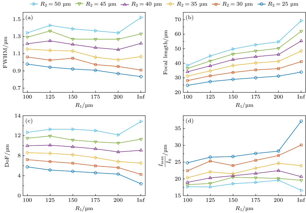
图 6 双凹型空气微透镜的厚度 t = 10 \mu\text{m} 时, (a) 焦斑横向 FWHM, (b) 焦距 FL, (c) 焦深 DoF 和 (d) 归一化焦点光强 I_{\text{max}}/I_0 随 R_1 和 R_2 的变化
