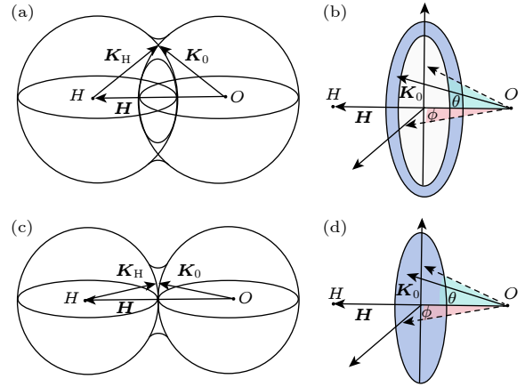
图 1 三维色散面及其截面的局部放大示意图 (a), (b) \theta_B < 90^\circ ; (c), (d) \theta_B \cong 90^\circ
