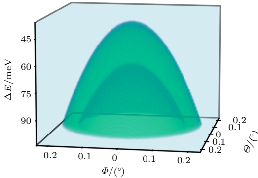
图 2 Si(800) 背散射的三维 DuMond 图
