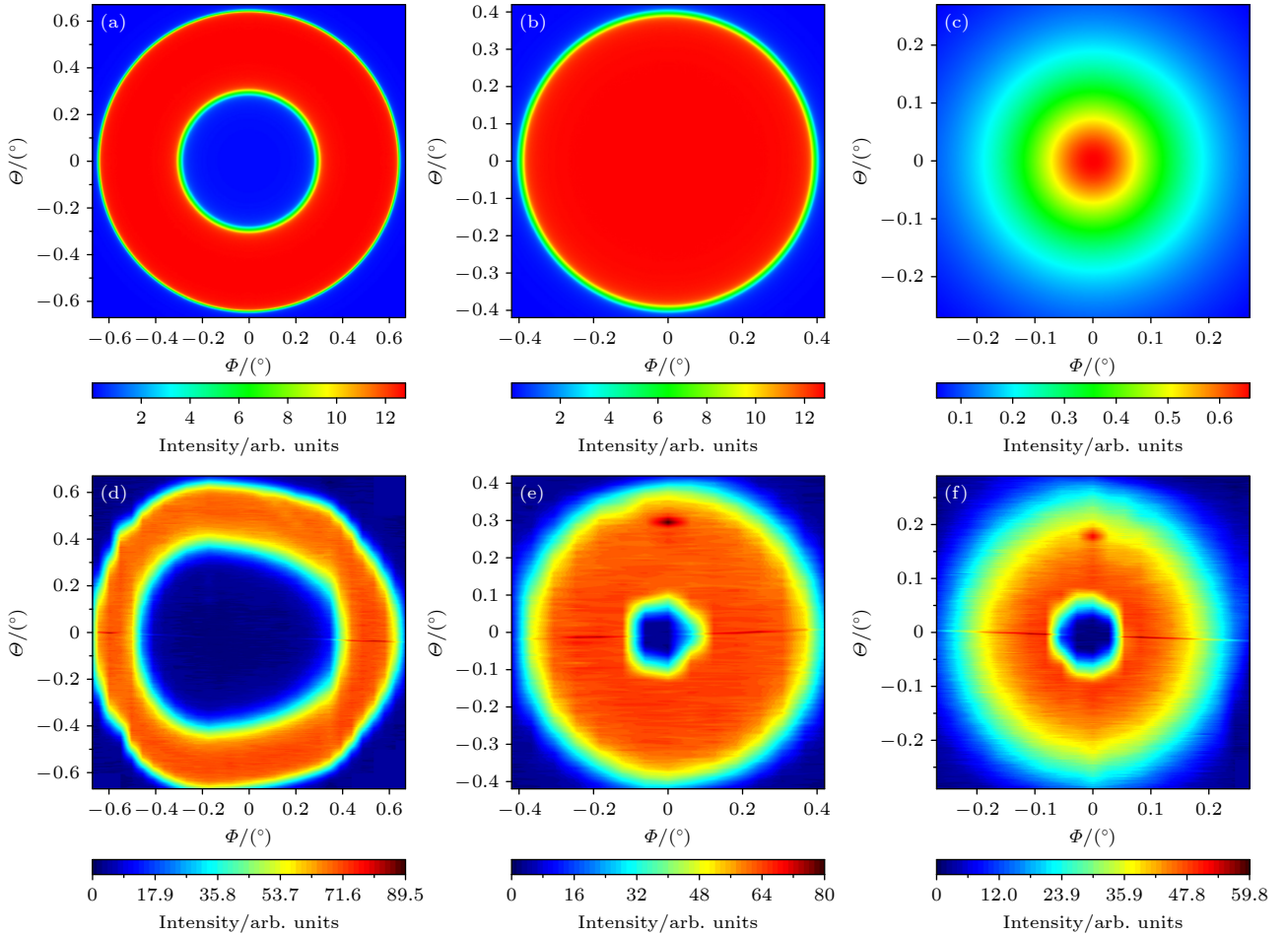
图 5 入射光带宽为 450 meV 时, 不同能量在 (\Theta, \Phi) 平面上的投影 (a)–(c) \delta E 分别为 400, 0 和 -200 meV 时的理论模拟结果; (d)–(f) 对应的实验测量结果
