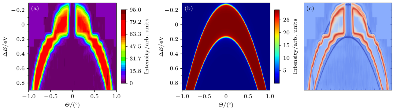
图 4 入射光带宽为 450 meV 时在 (\Delta E, \Theta) 平面上的投影 (a) 实验测量结果; (b) 理论模拟结果; (c) 实验与理论结果轮廓对比
