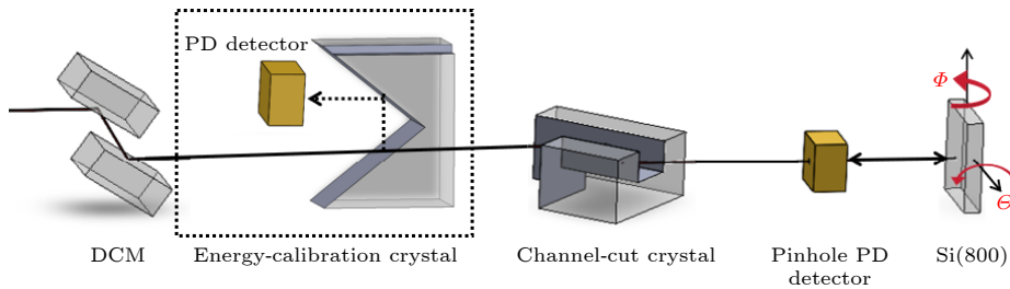
图 3 实验及能量校准系统光路示意图
